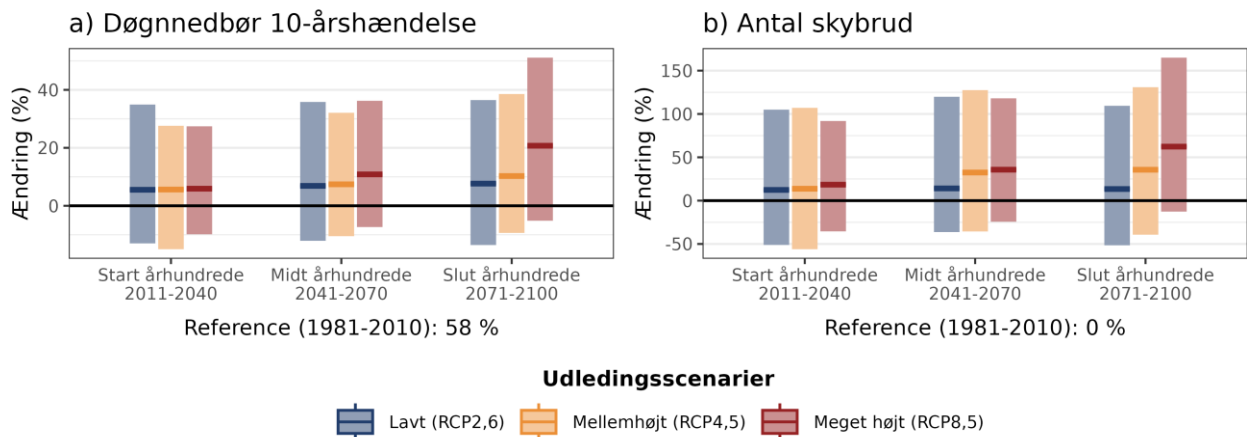
Figur 7. Procentvis ændring af a) 10-årshændelsen for døggnedbør og b) frekvensen af skybrud hen over året ift. 1981-2010 under forskellige udledningsscenerier i Sorø Kommune.
