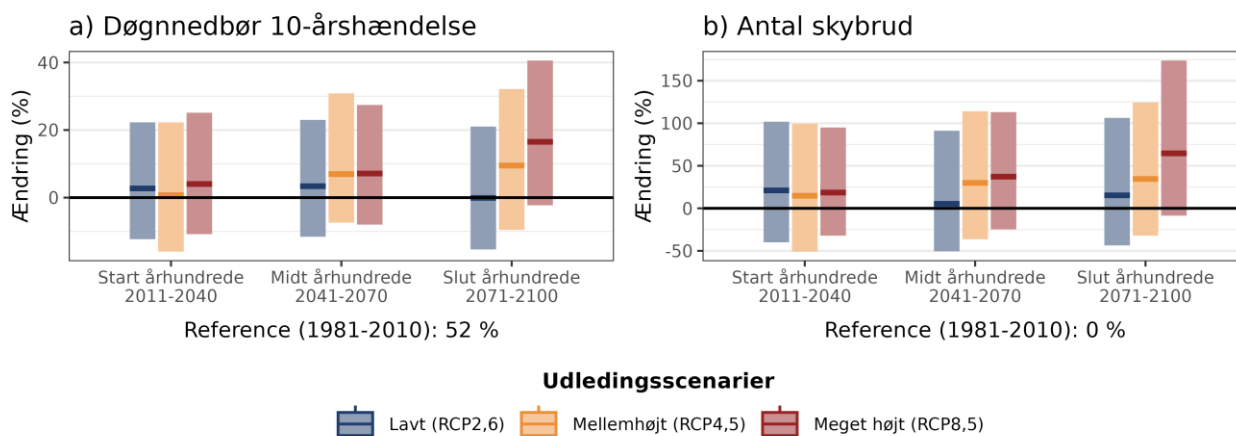
Figur 7. Procentvis ændring af a) 10-årshændelsen for døggnedbør og b) frekvensen af skybrud hen over året ift. 1981-2010 under forskellige udledningsscenerier i Skanderborg Kommune.
