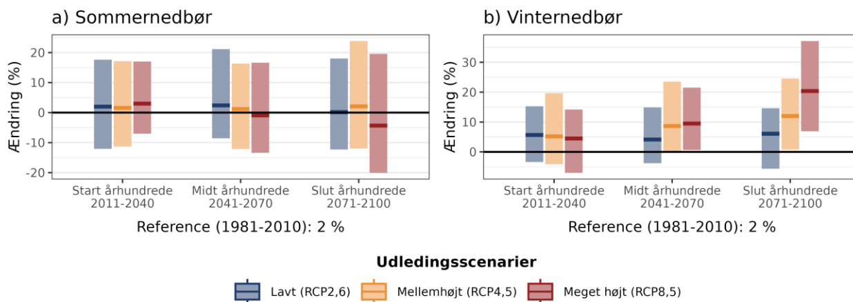
Figur 6. Procentvis ændring af middelnedbør a) om sommeren (jun-aug) og b) om vinteren (dec-feb) ift. referenceperioden 1981-2010 under forskellige udledningsscenerier i Skanderborg Kommune.
