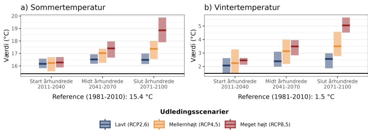
Figur 4. Fremtidens gennemsnitstemperatur for a) sommer (jun-aug) og b) vinter (dec-feb) under forskellige udledningsscenarioer i Skanderborg Kommune. Den sorte linje viser værdien for referenceperioden (1981-2010).
