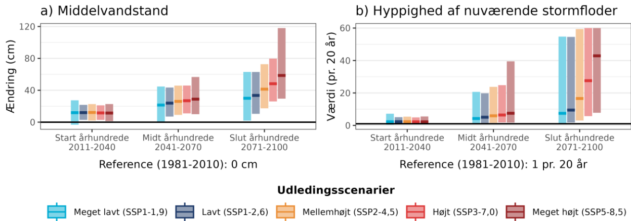
Figur 14. Fremtidens a) ændring i middelvandstand ift. referenceperioden 1981-2010 og b) hyppigheden af en nuværende 20-års stormflod for Sejerø Bugt under forskellige udledningsscenerier. Den sorte linje viser værdien for referenceperioden (1981-2010). Bemærk også at denne indikator maksimalt viser 60 stormfloder per 20 år, selv hvis de beregnede værdier bliver endnu højere.
