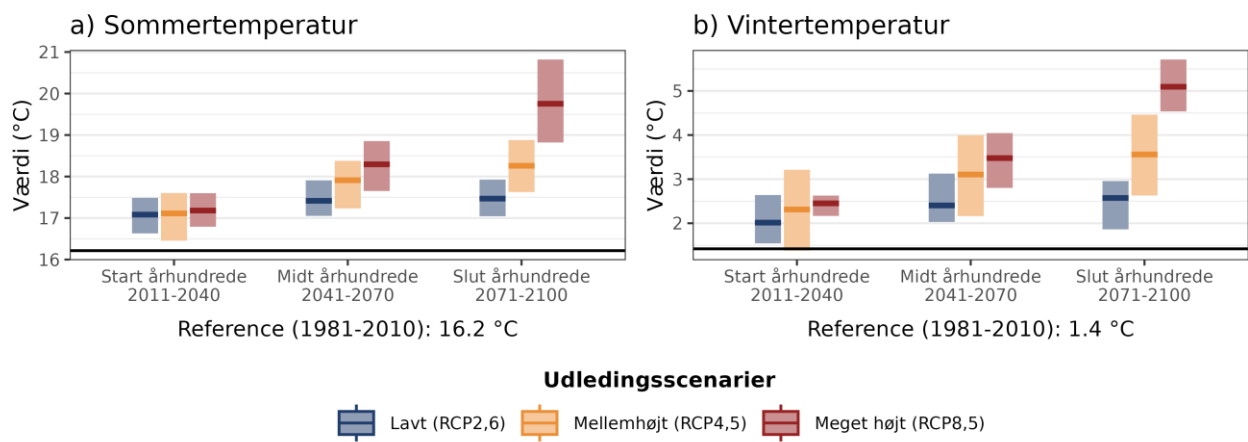
Figur 4. Fremtidens gennemsnitstemperatur for a) sommer (jun-aug) og b) vinter (dec-feb) under forskellige udledningsscenarier i Roskilde Kommune. Den sorte linje viser værdien for referenceperioden (1981-2010).
