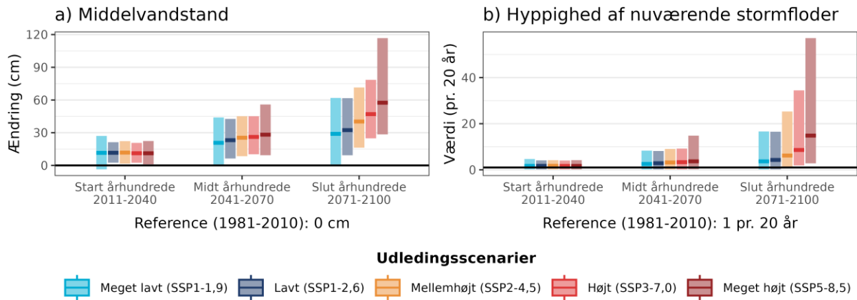
Figur 10. Fremtidens a) ændring i middelvandstand ift. referenceperioden 1981-2010 og b) hyppigheden af en nuværende 20-års stormflod for Roskilde Fjord under forskellige udledningsscenarioer. Den sorte linje viser værdien for referenceperioden (1981-2010). Bemærk også at denne indikator maksimalt viser 60 stormfloder per 20 år, selv hvis de beregnede værdier bliver endnu højere.
