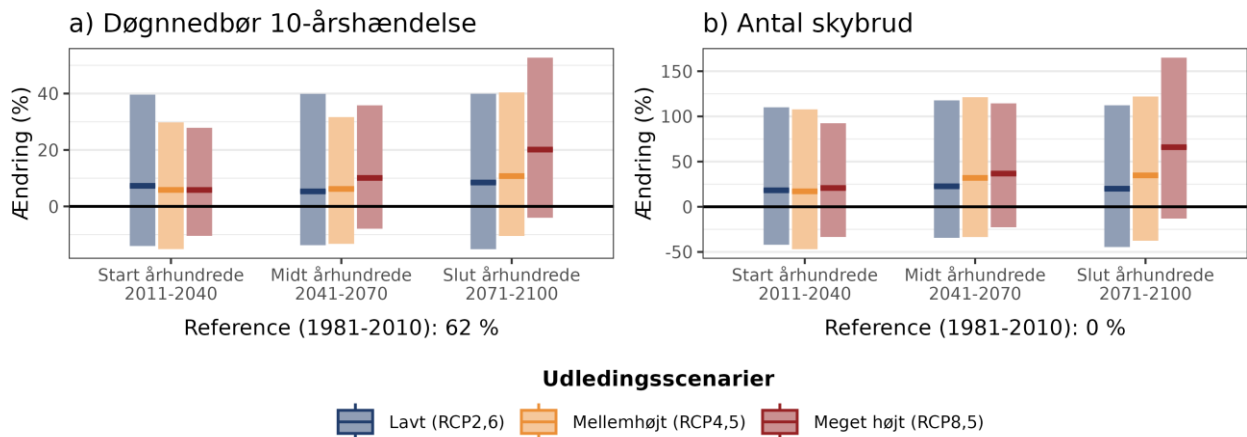
Figur 7. Procentvis ændring af a) 10-årshændelsen for døggnedbør og b) frekvensen af skybrud hen over året ift. 1981-2010 under forskellige udledningsscenerier i Roskilde Kommune.
