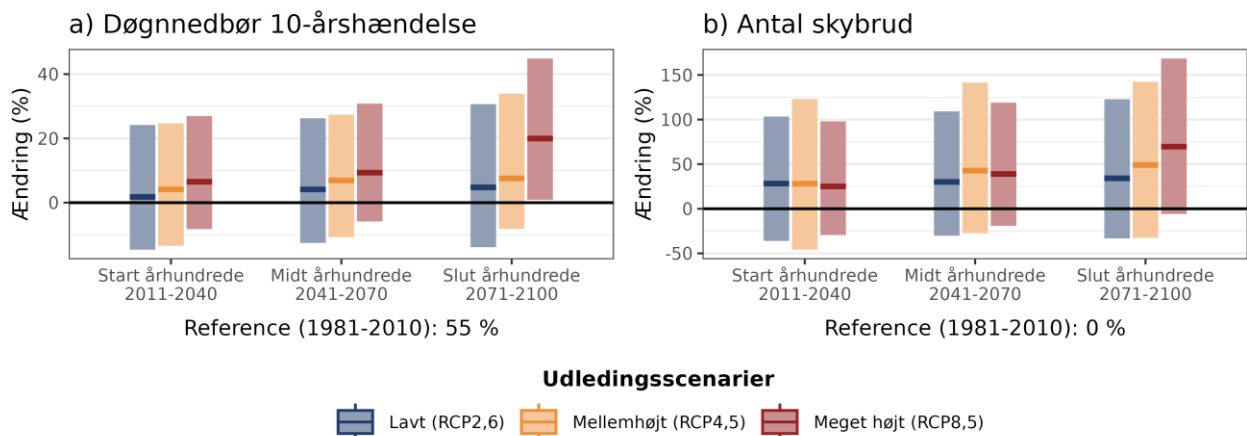
Figur 7. Procentvis ændring af a) 10-årshændelsen for døggnedbør og b) frekvensen af skybrud hen over året ift. 1981-2010 under forskellige udledningsscenarioer i Ringkøbing-Skjern Kommune.
