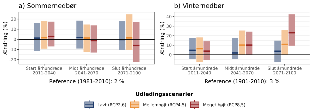
Figur 6. Procentvis ændring af middelnedbør a) om sommeren (jun-aug) og b) om vinteren (dec-feb) ift. referenceperioden 1981-2010 under forskellige udledningsscenarioer i Ringkøbing-Skjern Kommune.
