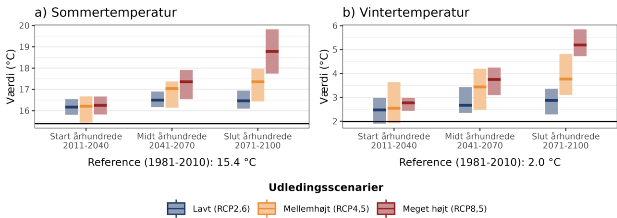
Figur 4. Fremtidens gennemsnitstemperatur for a) sommer (jun-aug) og b) vinter (dec-feb) under forskellige udledningsscenarioer i Ringkøbing-Skjern Kommune. Den sorte linje viser værdien for referenceperioden (1981-2010).
