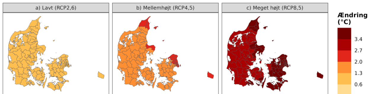
Figur 2. Ændring i gennemsnitstemperatur (°C) hen over året mellem 1981-2010 og 2071-2100 i a) lavt, b) mellemhøjt og c) højt udledningsscenario.
