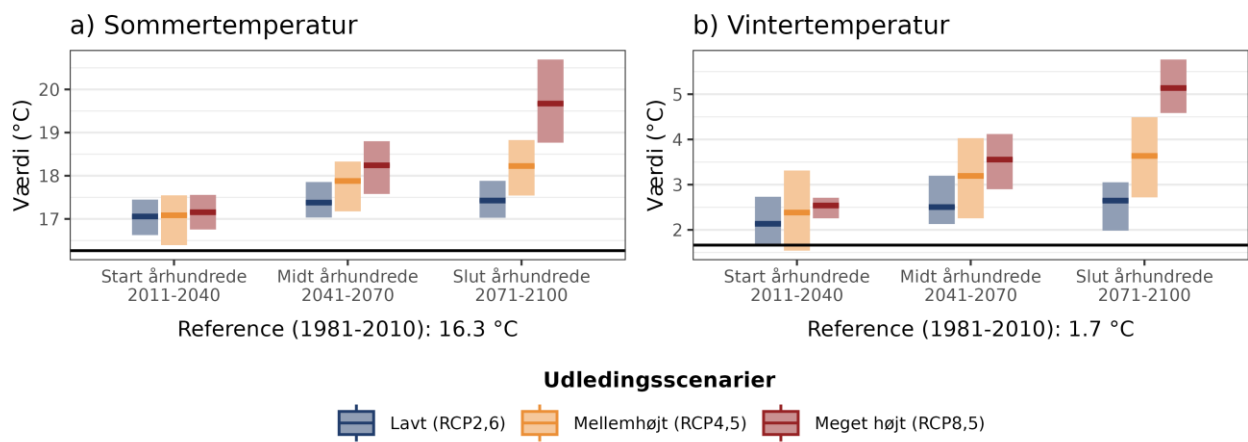
Figur 4. Fremtidens gennemsnitstemperatur for a) sommer (jun-aug) og b) vinter (dec-feb) under forskellige udledningsscenarioer i Odsherred Kommune. Den sorte linje viser værdien for referenceperioden (1981-2010).
