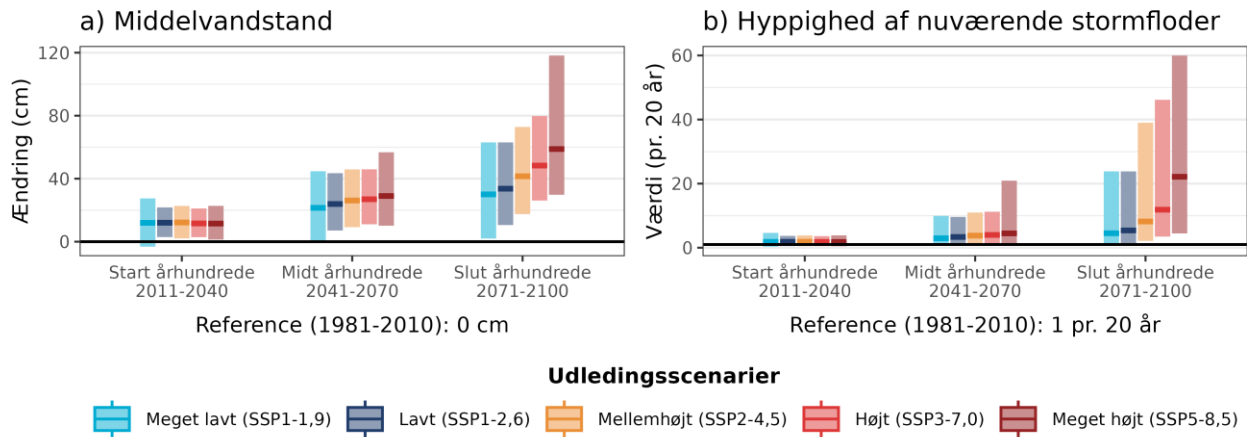
Figur 14. Fremtidens a) ændring i middelvandstand ift. referenceperioden 1981-2010 og b) hyppigheden af en nuværende 20-års stormflod for Isefjord under forskellige udledningsscenarioer. Den sorte linje viser værdien for referenceperioden (1981-2010). Bemærk også at denne indikator maksimalt viser 60 stormfloder per 20 år, selv hvis de beregnede værdier bliver endnu højere.
