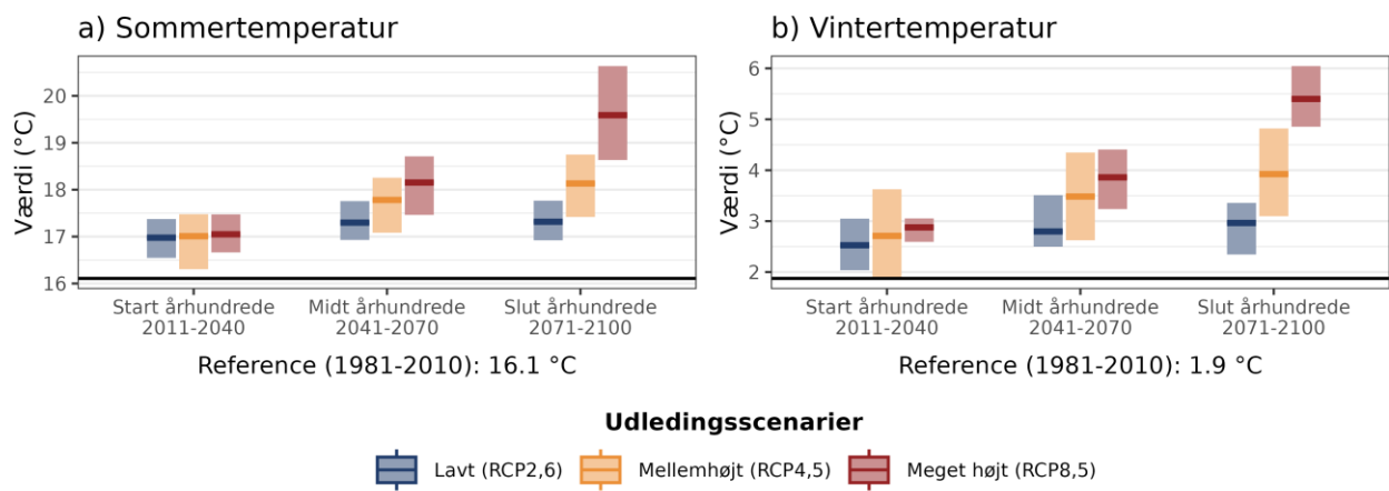
Figur 4. Fremtidens gennemsnitstemperatur for a) sommer (jun-aug) og b) vinter (dec-feb) under forskellige udledningsscenarier i Odense Kommune. Den sorte linje viser værdien for referenceperioden (1981-2010).
