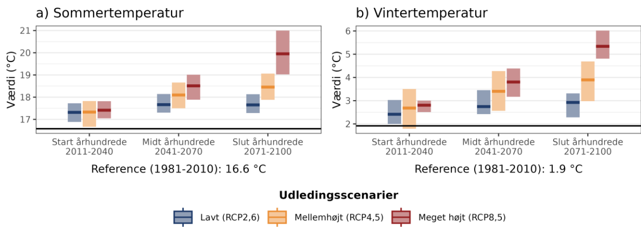
Figur 4. Fremtidens gennemsnitstemperatur for a) sommer (jun-aug) og b) vinter (dec-feb) under forskellige udledningsscenarioer i Lolland Kommune. Den sorte linje viser værdien for referenceperioden (1981-2010).
