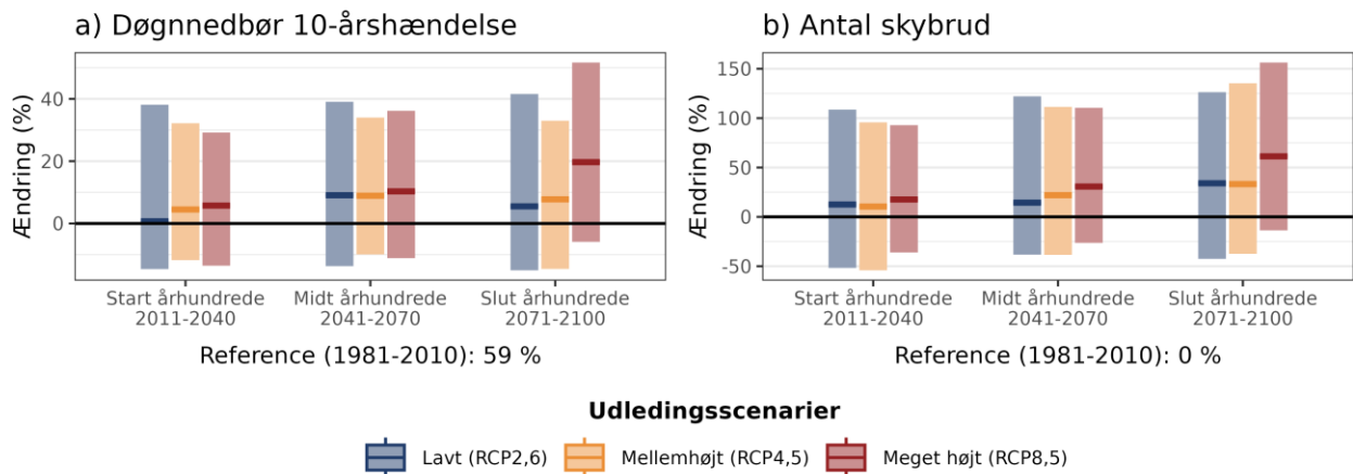
Figur 7. Procentvis ændring af a) 10-årshændelsen for døggnedbør og b) frekvensen af skybrud hen over året ift. 1981-2010 under forskellige udledningsscenerier i Langeland Kommune.
