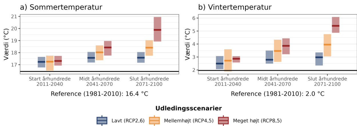
Figur 4. Fremtidens gennemsnitstemperatur for a) sommer (jun-aug) og b) vinter (dec-feb) under forskellige udledningsscenarioer i Langeland Kommune. Den sorte linje viser værdien for referenceperioden (1981-2010).
