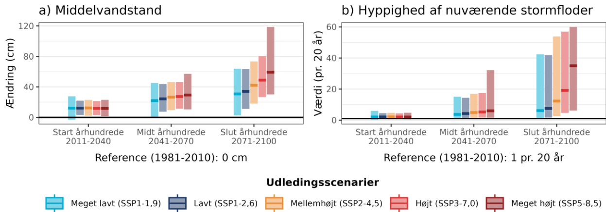
Figur 10. Fremtidens a) ændring i middelvandstand ift. referenceperioden 1981-2010 og b) hyppigheden af en nuværende 20-års stormflod for Storebælt nordøst under forskellige udledningsscenerier. Den sorte linje viser værdien for referenceperioden (1981-2010). Bemærk også at denne indikator maksimalt viser 60 stormfloder per 20 år, selv hvis de beregnede værdier bliver endnu højere.
