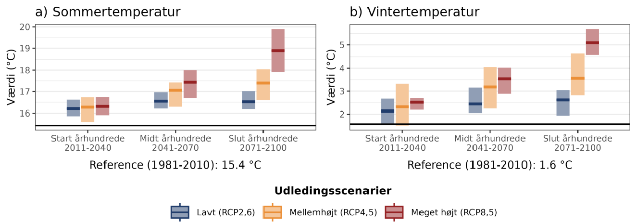
Figur 4. Fremtidens gennemsnitstemperatur for a) sommer (jun-aug) og b) vinter (dec-feb) under forskellige udledningsscenarioer i Horsens Kommune. Den sorte linje viser værdien for referenceperioden (1981-2010).
