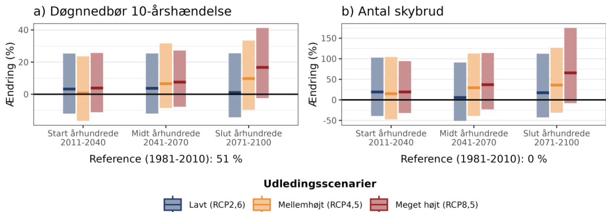
Figur 7. Procentvis ændring af a) 10-årshændelsen for døgnedbør og b) frekvensen af skybrud hen over året ift. 1981-2010 under forskellige udledningsscenerier i Horsens Kommune.
