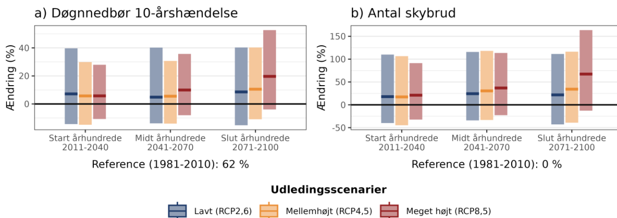
Figur 7. Procentvis ændring af a) 10-årshændelsen for døggnedbør og b) frekvensen af skybrud hen over året ift. 1981-2010 under forskellige udledningsscenarioer i Høje-Taastrup Kommune.
