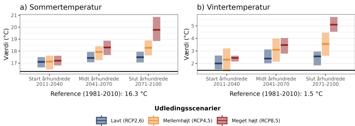
Figur 4. Fremtidens gennemsnitstemperatur for a) sommer (jun-aug) og b) vinter (dec-feb) under forskellige udledningsscenarioer i Høje-Taastrup Kommune. Den sorte linje viser værdien for referenceperioden (1981-2010).
