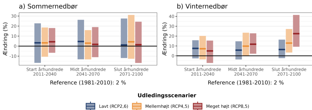
Figur 6. Procentvis ændring af middelnedbør a) om sommeren (jun-aug) og b) om vinteren (dec-feb) ift. referenceperioden 1981-2010 under forskellige udledningsscenarioer i Høje-Taastrup Kommune.
