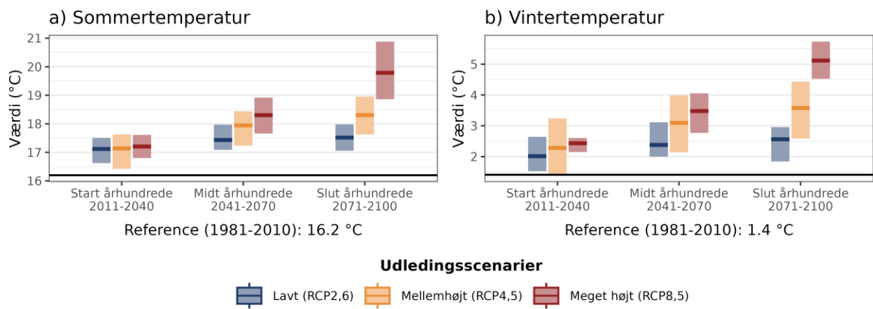
Figur 4. Fremtidens gennemsnitstemperatur for a) sommer (jun-aug) og b) vinter (dec-feb) under forskellige udledningsscenarier i Gribskov Kommune. Den sorte linje viser værdien for referenceperioden (1981-2010).
