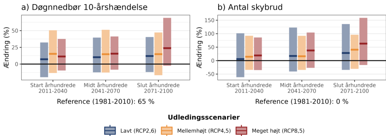
Figur 7. Procentvis ændring af a) 10-årshændelsen for døggnedbør og b) frekvensen af skybrud hen over året ift. 1981-2010 under forskellige udledningsscenerier i Bornholms Kommune.
