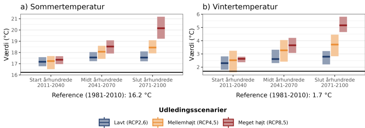
Figur 4. Fremtidens gennemsnitstemperatur for a) sommer (jun-aug) og b) vinter (dec-feb) under forskellige udledningsscenarioer i Bornholms Kommune. Den sorte linje viser værdien for referenceperioden (1981-2010).
