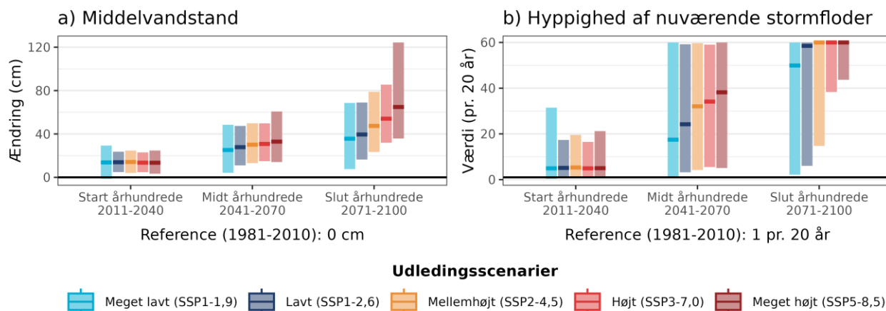
Figur 10. Fremtidens a) ændring i middelvandstand ift. referenceperioden 1981-2010 og b) hyppigheden af en nuværende 20-års stormflod for Bornholms kyst under forskellige udledningsscenarioer. Den sorte linje viser værdien for referenceperioden (1981-2010). Bemærk også at denne indikator maksimalt viser 60 stormfloder per 20 år, selv hvis de beregnede værdier bliver endnu højere.
