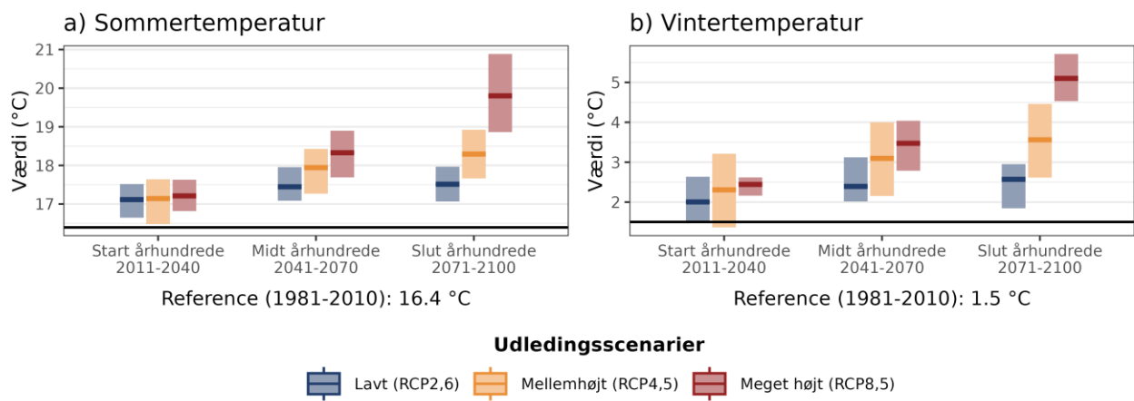
Figur 4. Fremtidens gennemsnitstemperatur for a) sommer (jun-aug) og b) vinter (dec-feb) under forskellige udledningsscenarioer i Albertslund Kommune. Den sorte linje viser værdien for referenceperioden (1981-2010).
