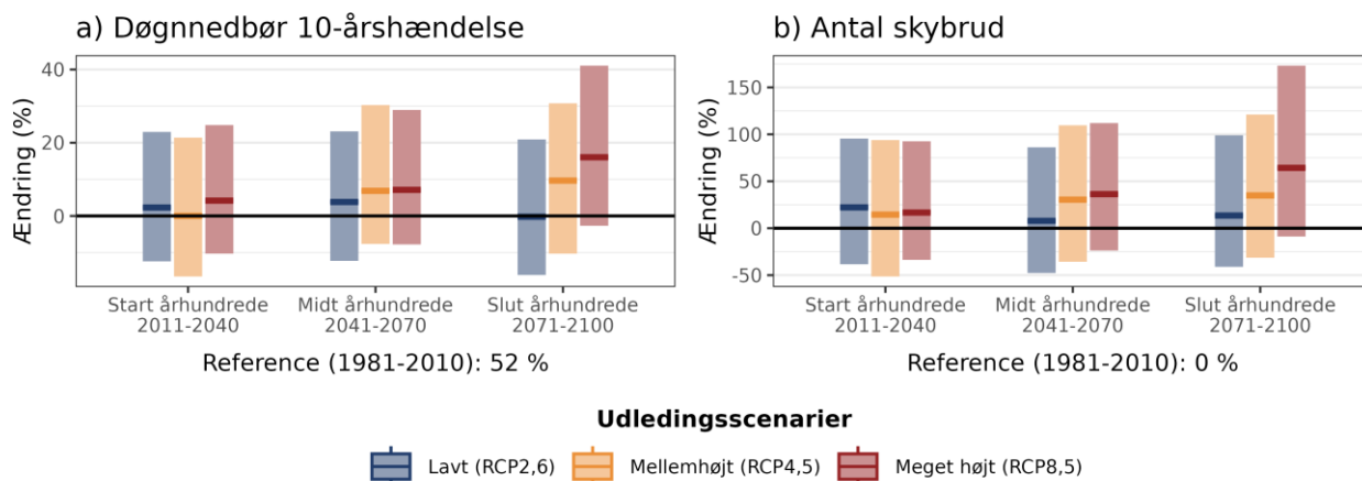
Figur 7. Procentvis ændring af a) 10-årshændelsen for døgnedbør og b) frekvensen af skybrud hen over året ift. 1981-2010 under forskellige udledningsscenarioer i Aarhus Kommune.
