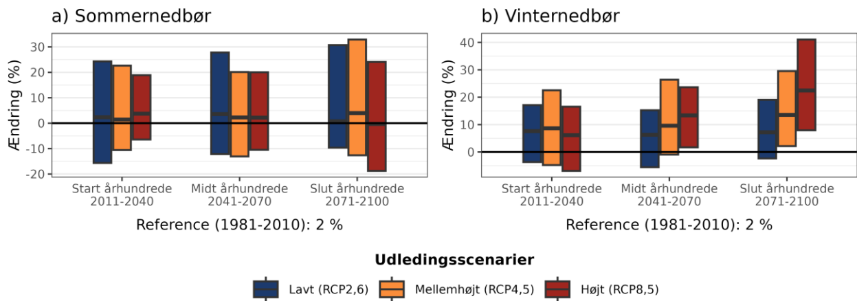
Figur 6. Procentvis ændring af middelnedbør a) om sommeren (jun-aug) og b) om vinteren (dec-feb) ift. referenceperioden 1981-2010 under forskellige udledningsscenerier i Vordingborg Kommune.
