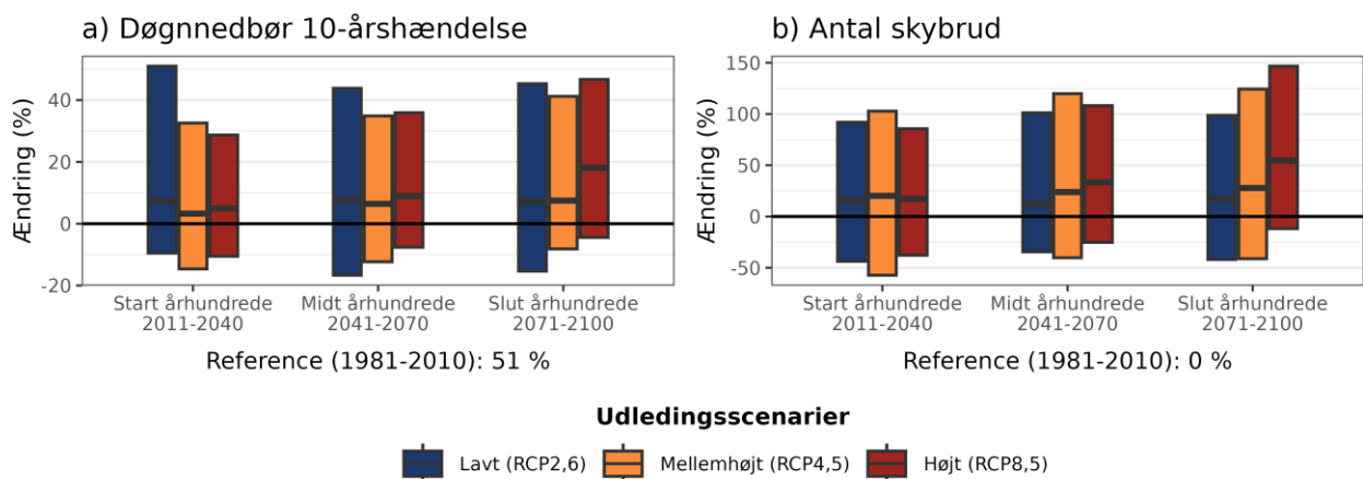
Figur 7. Procentvis ændring af a) 10-årshændelsen for døggnedbør og b) frekvensen af skybrud hen over året ift. 1981-2010 under forskellige udledningsscenerier i Vordingborg Kommune.
