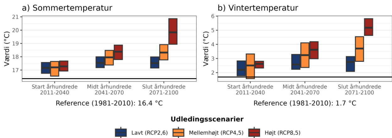
Figur 4. Fremtidens gennemsnitstemperatur for a) sommer (jun-aug) og b) vinter (dec-feb) under forskellige udledningsscenarioer i Vordingborg Kommune. Den sorte linje viser værdien for referenceperioden (1981-2010).
