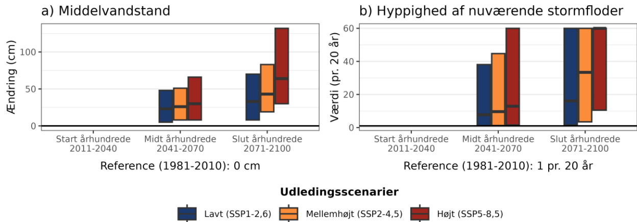
Figur 12. Fremtidens a) ændring i middelvandstand ift. referenceperioden 1981-2010 og b) hyppigheden af en nuværende 20-års stormflod for Falsters og Møns Østersøkyst under forskellige udledningsscenarioer. Den sorte linje viser værdien for referenceperioden (1981-2010). Bemærk også at denne indikator maksimalt viser 60 stormfloder per 20 år, selv hvis de beregnede værdier bliver endnu højere.
