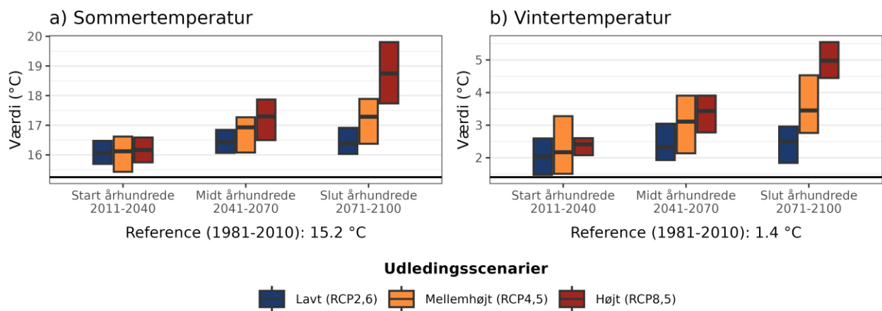
Figur 4. Fremtidens gennemsnitstemperatur for a) sommer (jun-aug) og b) vinter (dec-feb) under forskellige udledningsscenarioer i Viborg Kommune. Den sorte linje viser værdien for referenceperioden (1981-2010).
