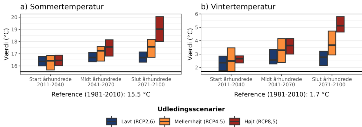
Figur 4. Fremtidens gennemsnitstemperatur for a) sommer (jun-aug) og b) vinter (dec-feb) under forskellige udledningsscenarioer i Vejen Kommune. Den sorte linje viser værdien for referenceperioden (1981-2010).
