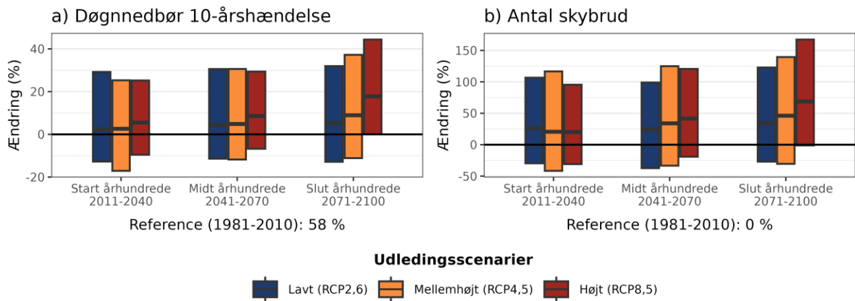
Figur 7. Procentvis ændring af a) 10-årshændelsen for døgnnedbør og b) frekvensen af skybrud hen over året ift. 1981-2010 under forskellige udledningsscenerier i Vejen Kommune.
