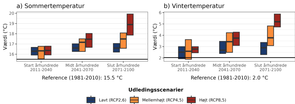
Figur 4. Fremtidens gennemsnitstemperatur for a) sommer (jun-aug) og b) vinter (dec-feb) under forskellige udledningsscenarioer i Varde Kommune. Den sorte linje viser værdien for referenceperioden (1981-2010).
