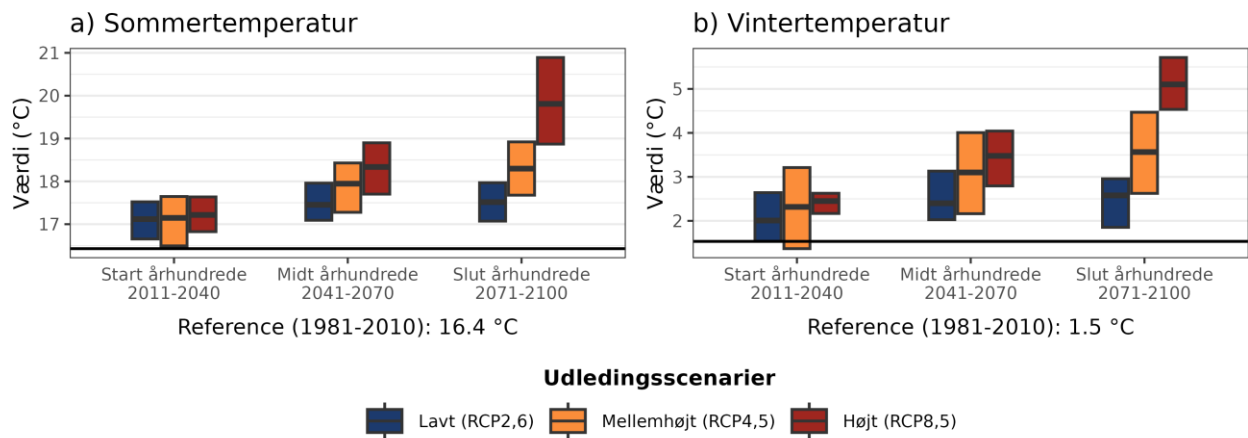
Figur 4. Fremtidens gennemsnitstemperatur for a) sommer (jun-aug) og b) vinter (dec-feb) under forskellige udledningsscenarioer i Vallensbæk Kommune. Den sorte linje viser værdien for referenceperioden (1981-2010).
