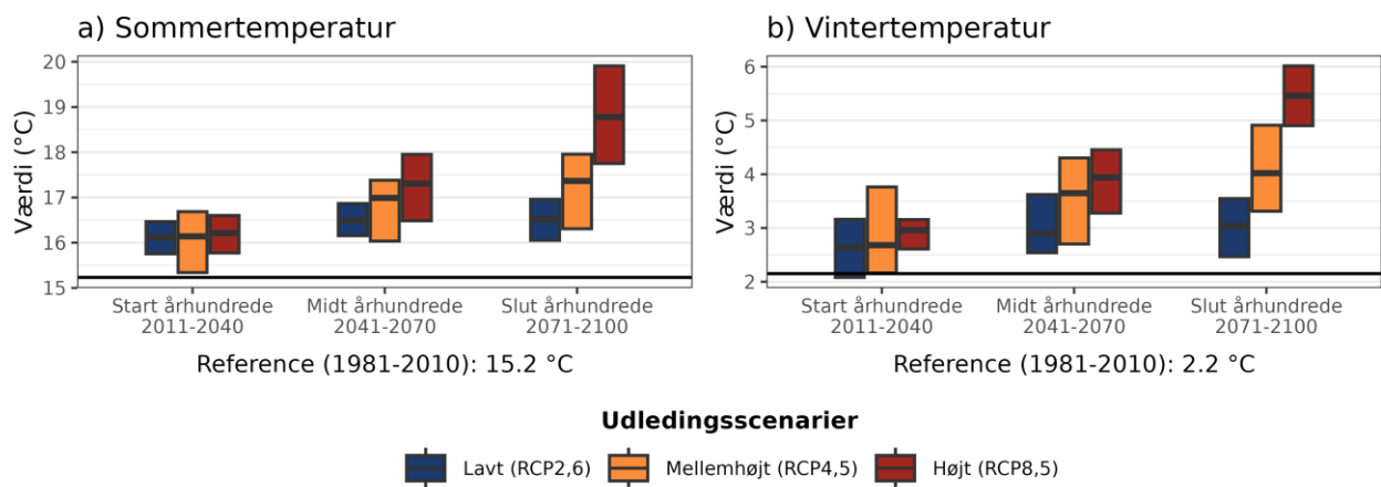
Figur 4. Fremtidens gennemsnitstemperatur for a) sommer (jun-aug) og b) vinter (dec-feb) under forskellige udledningsscenarioer i Thisted Kommune. Den sorte linje viser værdien for referenceperioden (1981-2010).
