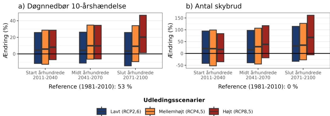
Figur 7. Procentvis ændring af a) 10-årshændelsen for døgnedbør og b) frekvensen af skybrud hen over året ift. 1981-2010 under forskellige udledningsscenerier i Thisted Kommune.
