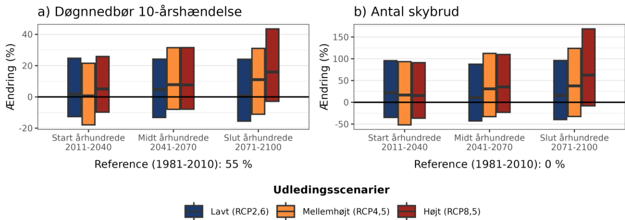
Figur 7. Procentvis ændring af a) 10-årshændelsen for døgnnedbør og b) frekvensen af skybrud hen over året ift. 1981-2010 under forskellige udledningsscenerier i Syddjurs Kommune.
