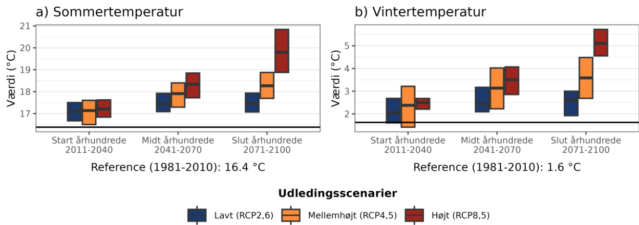
Figur 4. Fremtidens gennemsnitstemperatur for a) sommer (jun-aug) og b) vinter (dec-feb) under forskellige udledningsscenarioer i Stevns Kommune. Den sorte linje viser værdien for referenceperioden (1981-2010).
