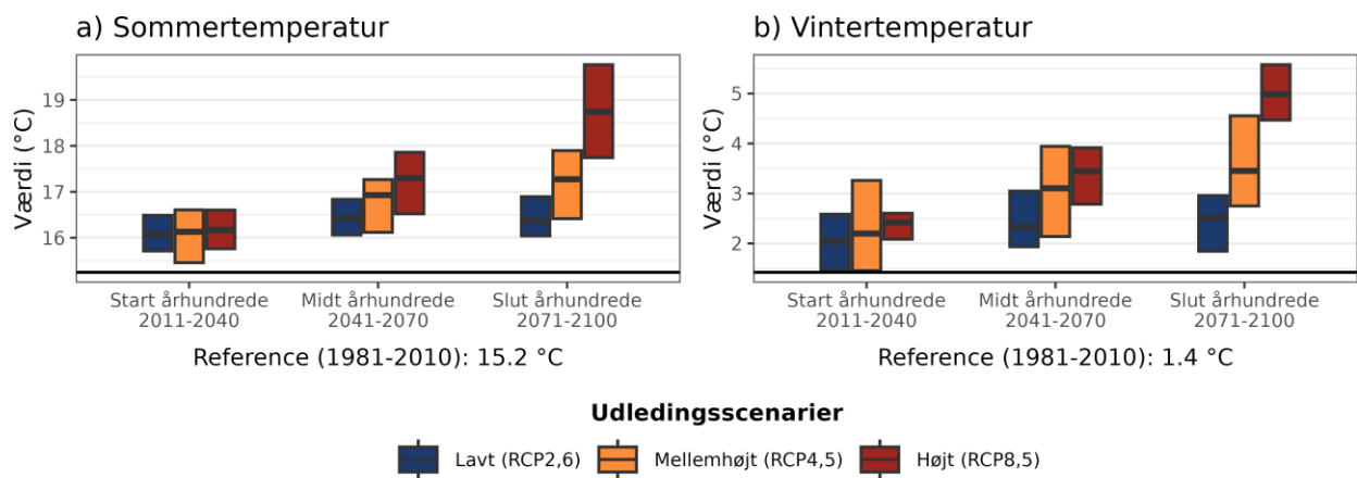
Figur 4. Fremtidens gennemsnitstemperatur for a) sommer (jun-aug) og b) vinter (dec-feb) under forskellige udledningsscenarioer i Silkeborg Kommune. Den sorte linje viser værdien for referenceperioden (1981-2010).
