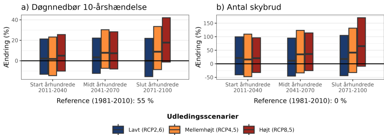
Figur 7. Procentvis ændring af a) 10-årshændelsen for døgngnedbør og b) frekvensen af skybrud hen over året ift. 1981-2010 under forskellige udledningsscenerier i Silkeborg Kommune.
