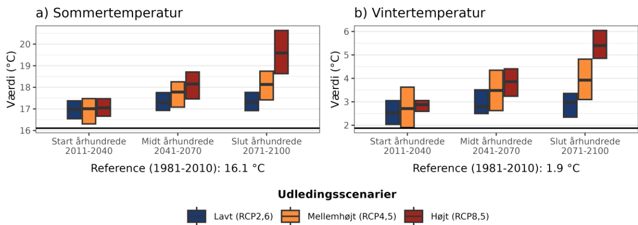
Figur 4. Fremtidens gennemsnitstemperatur for a) sommer (jun-aug) og b) vinter (dec-feb) under forskellige udledningsscenarioer i Odense Kommune. Den sorte linje viser værdien for referenceperioden (1981-2010).
