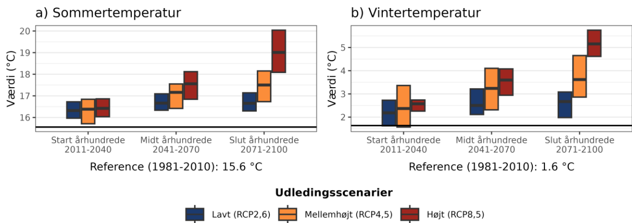
Figur 4. Fremtidens gennemsnitstemperatur for a) sommer (jun-aug) og b) vinter (dec-feb) under forskellige udledningsscenarioer i Odder Kommune. Den sorte linje viser værdien for referenceperioden (1981-2010).
