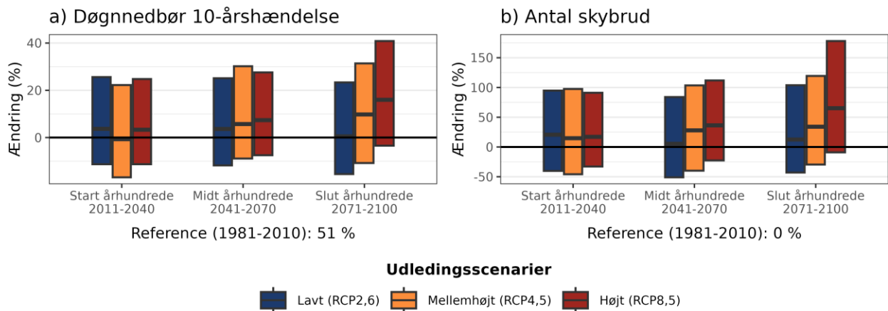
Figur 7. Procentvis ændring af a) 10-årshændelsen for døgnedbør og b) frekvensen af skybrud hen over året ift. 1981-2010 under forskellige udledningsscenerier i Odder Kommune.
