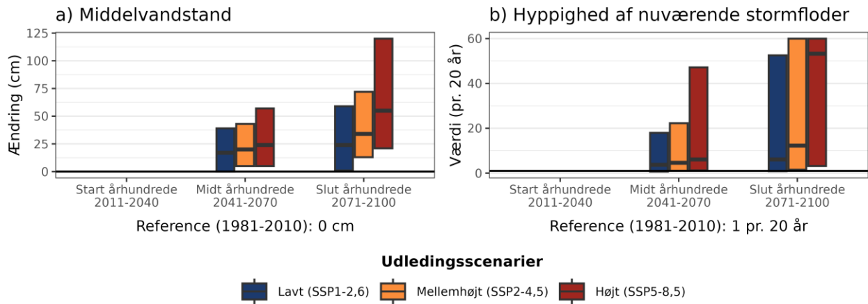
Figur 10. Fremtidens a) ændring i middelvandstand ift. referenceperioden 1981-2010 og b) hyppigheden af en nuværende 20-års stormflod for Ålborg Bugt under forskellige udledningsscenerier. Den sorte linje viser værdien for referenceperioden (1981-2010). Bemærk også at denne indikator maksimalt viser 60 stormfloder per 20 år, selv hvis de beregnede værdier bliver endnu højere.
