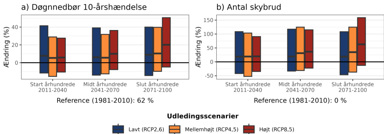
Figur 7. Procentvis ændring af a) 10-årshændelsen for døggnedbør og b) frekvensen af skybrud hen over året ift. 1981-2010 under forskellige udledningsscenerier i Køge Kommune.
