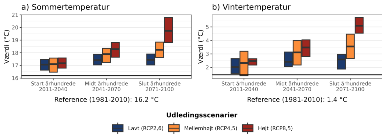
Figur 4. Fremtidens gennemsnitstemperatur for a) sommer (jun-aug) og b) vinter (dec-feb) under forskellige udledningsscenarioer i Køge Kommune. Den sorte linje viser værdien for referenceperioden (1981-2010).
