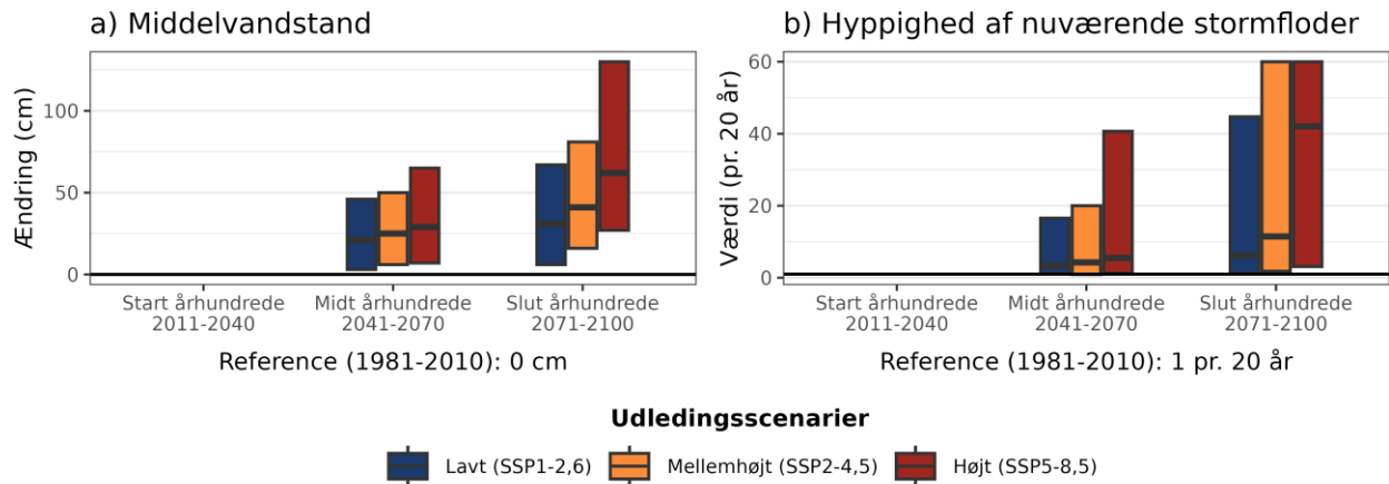
Figur 12. Fremtidens a) ændring i middelvandstand ift. referenceperioden 1981-2010 og b) hyppigheden af en nuværende 20-års stormflod for Sejerø Bugt under forskellige udledningsscenarioer. Den sorte linje viser værdien for referenceperioden (1981-2010). Bemærk også at denne indikator maksimalt viser 60 stormfloder per 20 år, selv hvis de beregnede værdier bliver endnu højere.
