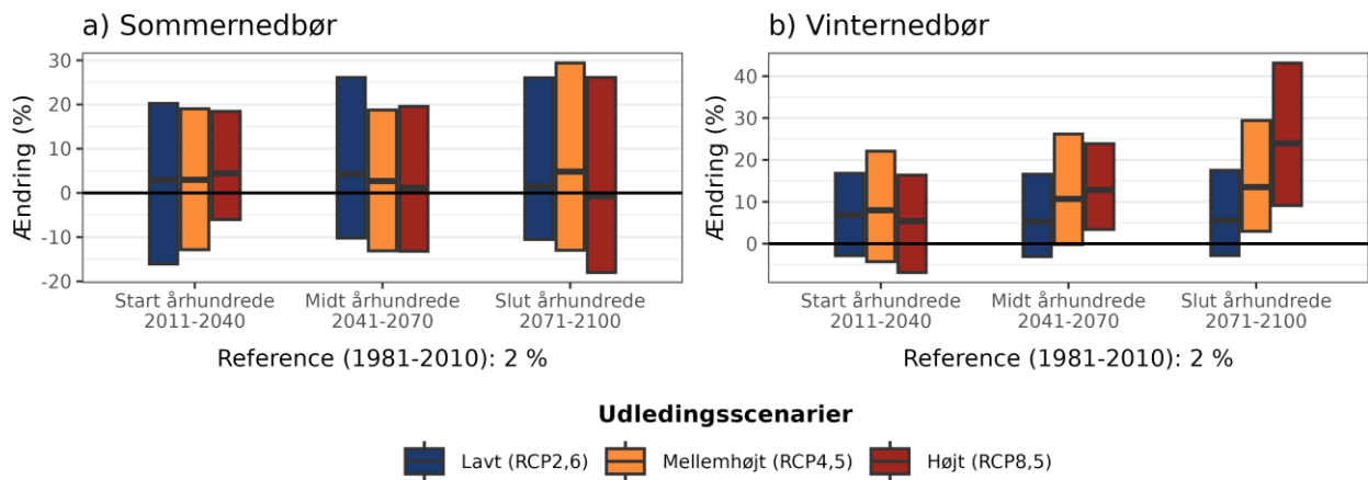
Figur 6. Procentvis ændring af middelnedbør a) om sommeren (jun-aug) og b) om vinteren (dec-feb) ift. referenceperioden 1981-2010 under forskellige udledningsscenarioer i Kalundborg Kommune.
