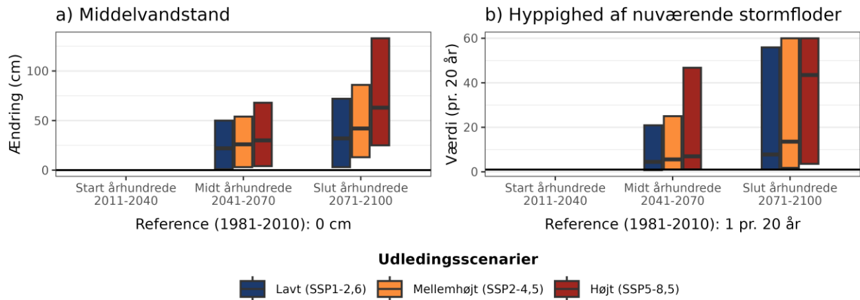
Figur 10. Fremtidens a) ændring i middelvandstand ift. referenceperioden 1981-2010 og b) hyppigheden af en nuværende 20-års stormflod for Storebælt nordøst under forskellige udledningsscenarioer. Den sorte linje viser værdien for referenceperioden (1981-2010). Bemærk også at denne indikator maksimalt viser 60 stormfloder per 20 år, selv hvis de beregnede værdier bliver endnu højere.
