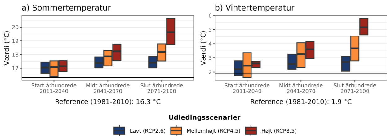
Figur 4. Fremtidens gennemsnitstemperatur for a) sommer (jun-aug) og b) vinter (dec-feb) under forskellige udledningsscenarioer i Kalundborg Kommune. Den sorte linje viser værdien for referenceperioden (1981-2010).
