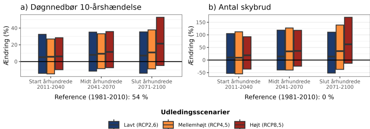
Figur 7. Procentvis ændring af a) 10-årshændelsen for døggnedbør og b) frekvensen af skybrud hen over året ift. 1981-2010 under forskellige udledningsscenarioer i Kalundborg Kommune.
