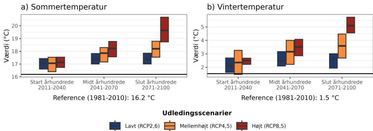
Figur 4. Fremtidens gennemsnitstemperatur for a) sommer (jun-aug) og b) vinter (dec-feb) under forskellige udledningsscenarioer i Holbæk Kommune. Den sorte linje viser værdien for referenceperioden (1981-2010).
