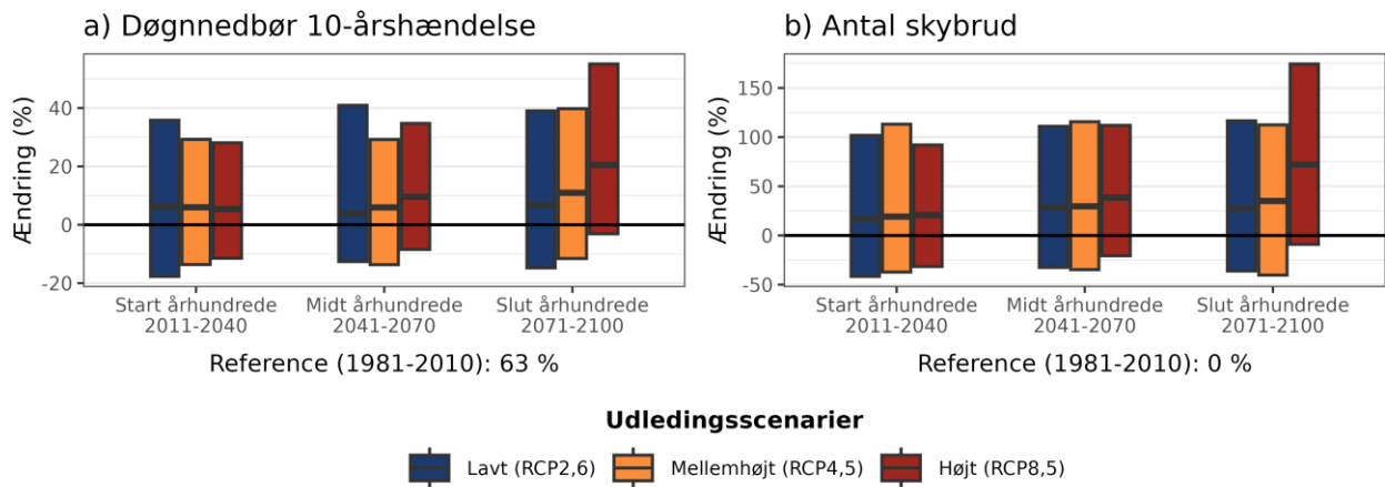
Figur 7. Procentvis ændring af a) 10-årshændelsen for døgnnedbør og b) frekvensen af skybrud hen over året ift. 1981-2010 under forskellige udledningsscenerier i Hørsholm Kommune.
