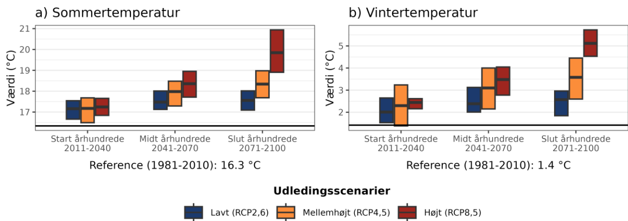
Figur 4. Fremtidens gennemsnitstemperatur for a) sommer (jun-aug) og b) vinter (dec-feb) under forskellige udledningsscenarioer i Hørsholm Kommune. Den sorte linje viser værdien for referenceperioden (1981-2010).
