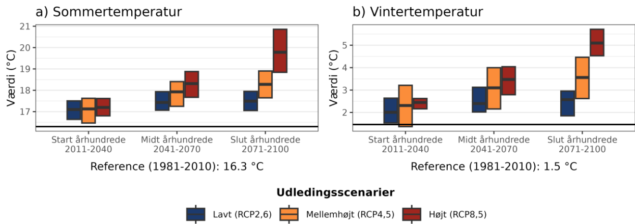
Figur 4. Fremtidens gennemsnitstemperatur for a) sommer (jun-aug) og b) vinter (dec-feb) under forskellige udledningsscenarier i Høje-Taastrup Kommune. Den sorte linje viser værdien for referenceperioden (1981-2010).
