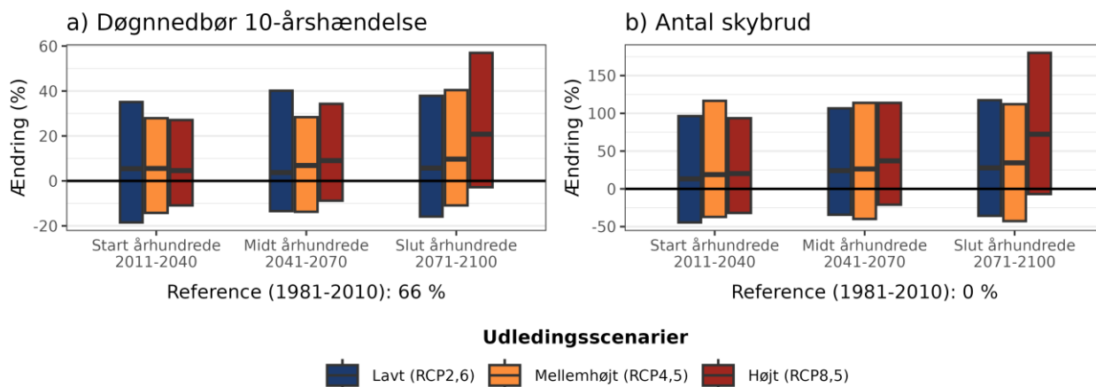
Figur 7. Procentvis ændring af a) 10-årshændelsen for døgnnedbør og b) frekvensen af skybrud hen over året ift. 1981-2010 under forskellige udledningsscenarioer i Helsingør Kommune.
