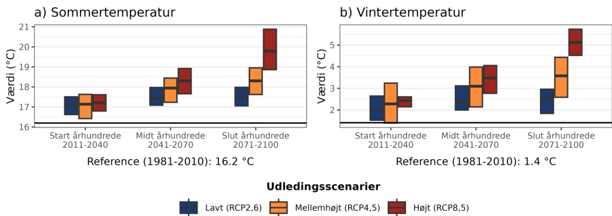
Figur 4. Fremtidens gennemsnitstemperatur for a) sommer (jun-aug) og b) vinter (dec-feb) under forskellige udledningsscenarioer i Gribskov Kommune. Den sorte linje viser værdien for referenceperioden (1981-2010).
