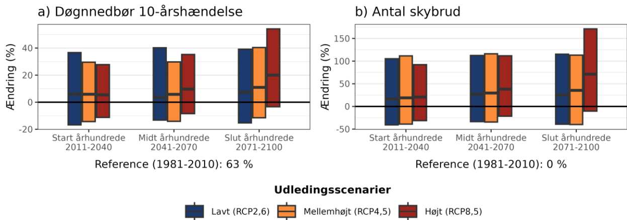
Figur 7. Procentvis ændring af a) 10-årshændelsen for døgnnedbør og b) frekvensen af skybrud hen over året ift. 1981-2010 under forskellige udledningsscenerier i Furesø Kommune.
