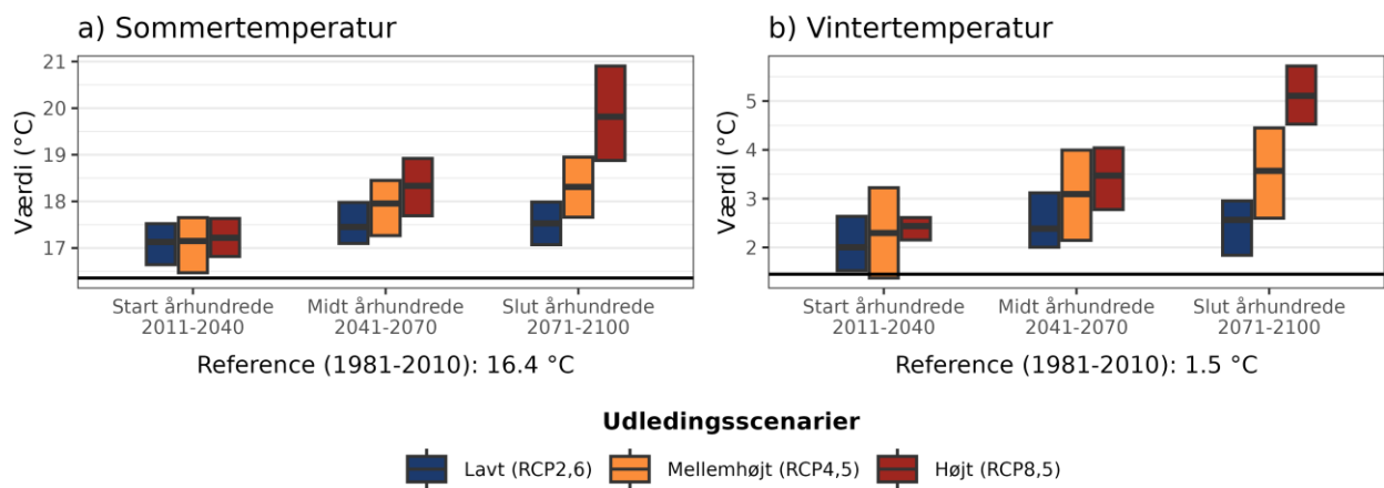
Figur 4. Fremtidens gennemsnitstemperatur for a) sommer (jun-aug) og b) vinter (dec-feb) under forskellige udledningsscenarioer i Furesø Kommune. Den sorte linje viser værdien for referenceperioden (1981-2010).
