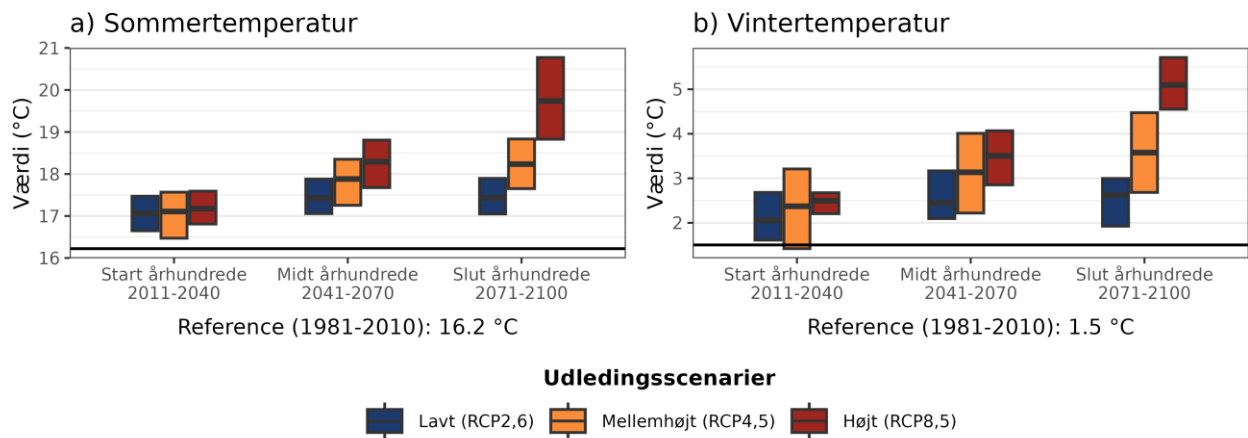
Figur 4. Fremtidens gennemsnitstemperatur for a) sommer (jun-aug) og b) vinter (dec-feb) under forskellige udledningsscenarioer i Faxe Kommune. Den sorte linje viser værdien for referenceperioden (1981-2010).
