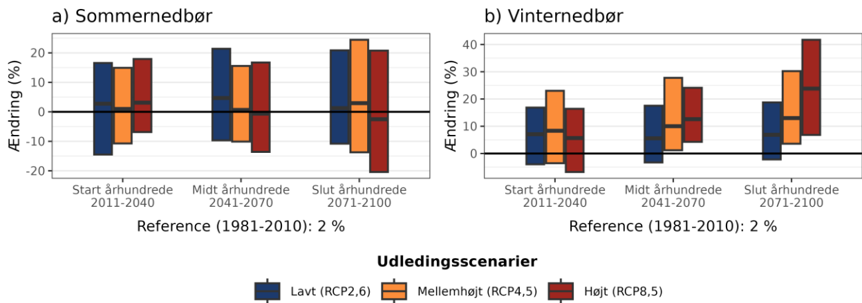
Figur 6. Procentvis ændring af middelnedbør a) om sommeren (jun-aug) og b) om vinteren (dec-feb) ift. referenceperioden 1981-2010 under forskellige udledningsscenerier i Faaborg-Midtfyn Kommune.
