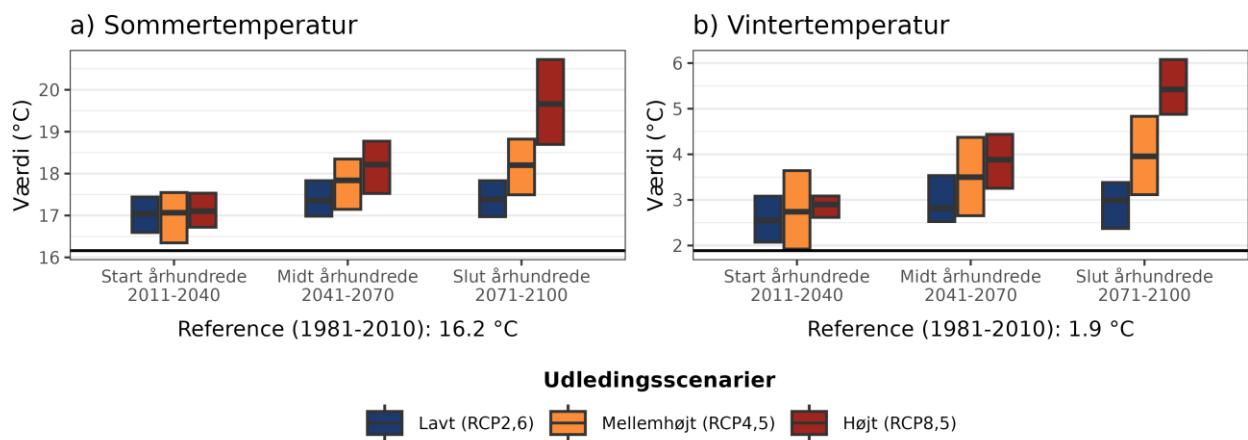
Figur 4. Fremtidens gennemsnitstemperatur for a) sommer (jun-aug) og b) vinter (dec-feb) under forskellige udledningsscenarioer i Faaborg-Midtfyn Kommune. Den sorte linje viser værdien for referenceperioden (1981-2010).
