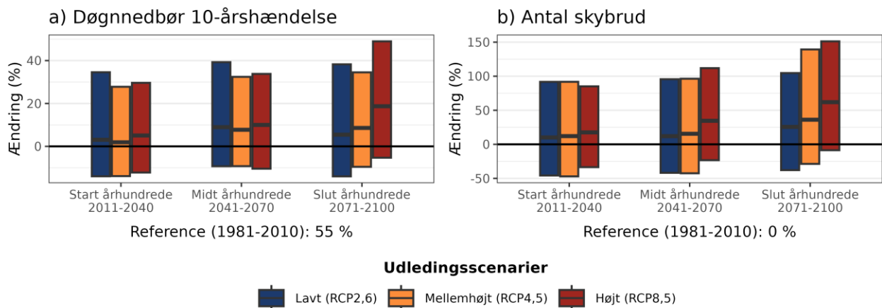
Figur 7. Procentvis ændring af a) 10-årshændelsen for døggnedbør og b) frekvensen af skybrud hen over året ift. 1981-2010 under forskellige udledningsscenerier i Faaborg-Midtfyn Kommune.
