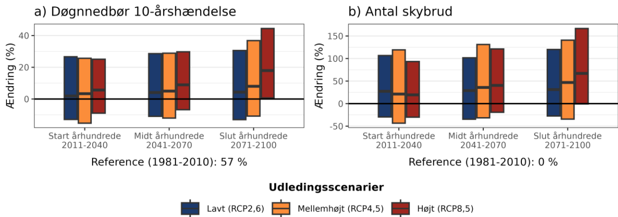
Figur 7. Procentvis ændring af a) 10-årshændelsen for døgnedbør og b) frekvensen af skybrud hen over året ift. 1981-2010 under forskellige udledningsscenerier i Esbjerg Kommune.
