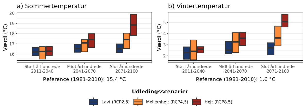
Figur 4. Fremtidens gennemsnitstemperatur for a) sommer (jun-aug) og b) vinter (dec-feb) under forskellige udledningsscenarioer i Billund Kommune. Den sorte linje viser værdien for referenceperioden (1981-2010).
