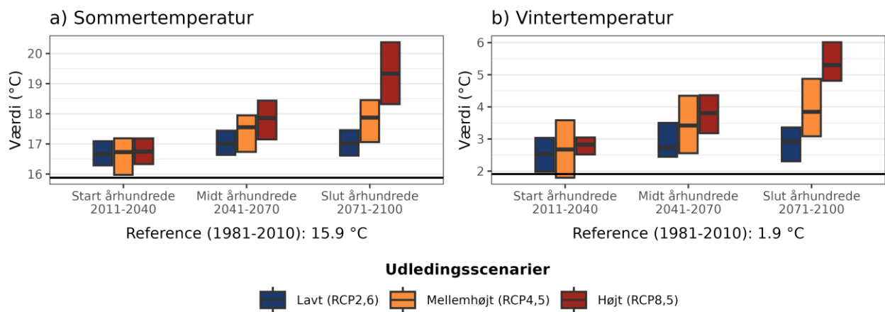
Figur 4. Fremtidens gennemsnitstemperatur for a) sommer (jun-aug) og b) vinter (dec-feb) under forskellige udledningsscenarioer i Aabenraa Kommune. Den sorte linje viser værdien for referenceperioden (1981-2010).
