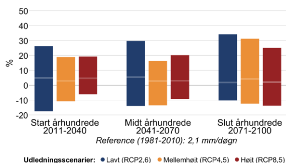
Figur 6 Procentvis ændring af middelnedbør mellem 1981-2010 og fremtidsperioderne 2011-2040, 2041-2070 og 2071-2100 under forskellige udledningsscenarier i Solrød Kommune. Til venstre sommer (jun-aug), til højre vinter (dec-feb).
