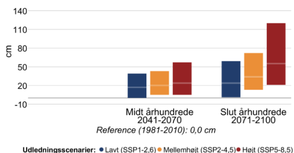
Figur 10 Ændring i middelvandstand (venstre) og hyppigheden af stormflod for Ålborg Bugt i fremtidsperioderne 2041-2070 og 2071-2100 under forskellige udledningsscenarier. Den grå linje viser referenceværdien for nutiden (1981-2010). En stormflod
