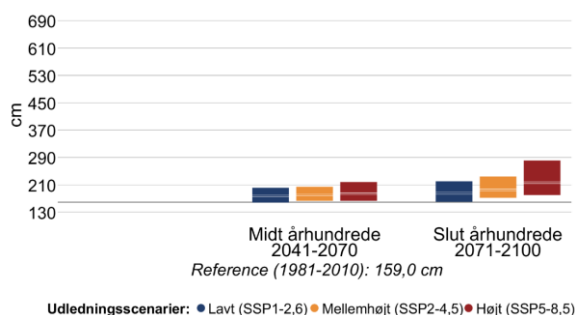
Figur 13 Højden af 20- (venstre) og 100-års (højre) stormflodshændelser for Randers Fjord og Mariager Fjord i fremtidsperioderne 2041-2070 og 2071-2100 under forskellige udledningsscenarier. Den grå linje viser referenceværdien for nutiden (1981-2010).
