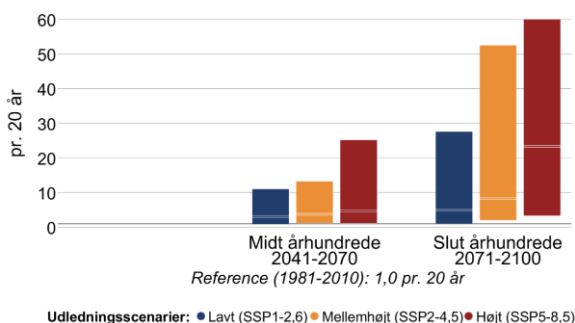
Figur 12 Ændring i middelvandstand (venstre) og hyppigheden af stormflod for Randers Fjord og Mariager Fjord i fremtidsperioderne 2041-2070 og 2071-2100 under forskellige udledningsscenarier. Den grå linje viser referenceværdien for nutiden (1981-2010). En stormflod defineres her som en forhøjet vandstand, der statistisk set kun forekommer én gang hvert 20. år i perioden 1981-2010. Bemærk også at denne indikator kappes ved 60 stormfloder per 20 år.
