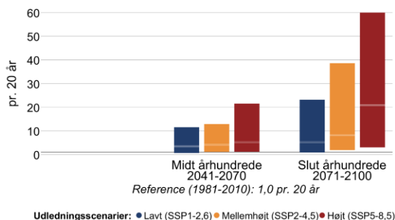
Figur 14 Ændring i middelvandstand (venstre) og hyppigheden af stormflod for Djurslands østkyst og Anholt i fremtidsperioderne 2041-2070 og 2071-2100 under forskellige udledningsscenarier. Den grå linje viser referenceværdien for nutiden (1981-2010). En stormflod defineres her som en forhøjet vandstand, der statistisk set kun forekommer én gang hvert 20. år i perioden 1981-2010. Bemærk også at denne indikator kappes ved 60 stormfloder per 20 år.
