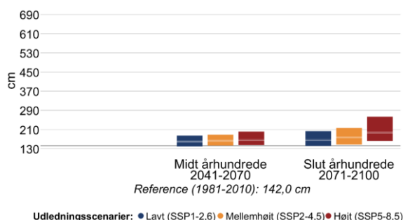
Figur 11 Højden af 20- (venstre) og 100-års (højre) stormflodshændelser for Ålborg Bugt i fremtidsperioderne 2041-2070 og 2071-2100 under forskellige udledningsscenarier. Den grå linje viser referenceværdien for nutiden (1981-2010).
