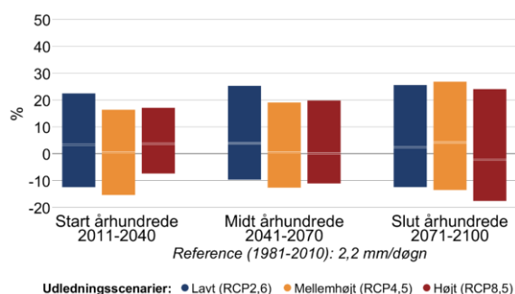
Figur 6 Procentvis ændring af middelnedbør mellem 1981-2010 og fremtidsperioderne 2011-2040, 2041-2070 og 2071-2100 under forskellige udledningsscenarier i Norddjurs Kommune. Til venstre sommer (jun-aug), til højre vinter (dec-feb).
