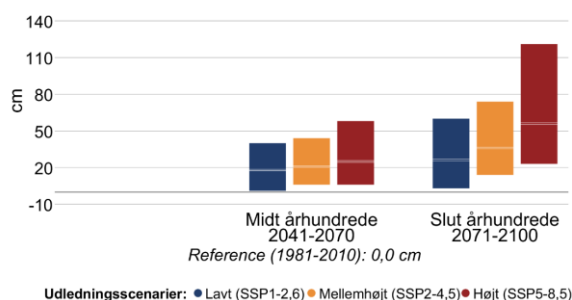
Figur 12 Ændring i middelvandstand (venstre) og hyppigheden af stormflod for Randers Fjord og Mariager Fjord i fremtidsperioderne 2041-2070 og 2071-2100 under forskellige udledningsscenarier. Den grå linje viser referenceværdien for nutiden (1981-2010). En stormflod defineres her som en forhøjet vandstand, der statistisk set kun forekommer én gang hvert 20. år i perioden 1981-2010. Bemærk også at denne indikator kappes ved 60 stormfloder per 20 år.
