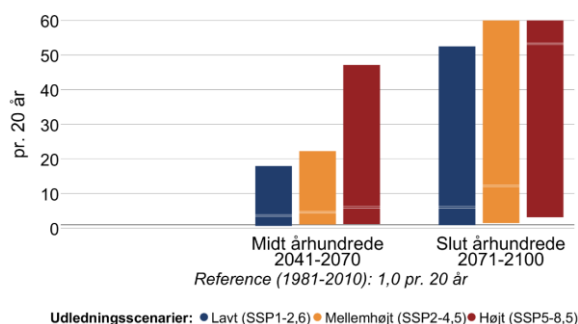
Figur 10 Ændring i middelvandstand (venstre) og hyppigheden af stormflod for Ålborg Bugt i fremtidsperioderne 2041-2070 og 2071-2100 under forskellige udledningsscenarier. Den grå linje viser referenceværdien for nutiden (1981-2010). En stormflod
