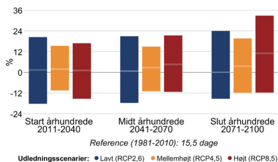
Figur 8 Procentvis ændring af tørre dage om sommeren (jun-aug) mellem 1981-2010 og fremtidsperioderne 2011-2040, 2041-2070 og 2071-2100 under forskellige udledningsscenarier i Norddjurs Kommune. Til venstre antallet af tørre dage med mindre end 1 mm nedbør, til højre længden af den længste sammenhængende tørre periode.
