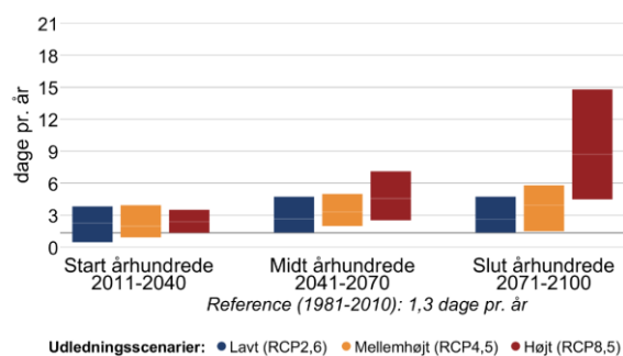
Figur 3 Ændring af gennemsnitstemperatur og antallet af hedebølgedage hen over året mellem 1981-2010 og fremtidsperioderne 2011-2040, 2041-2070 og 2071-2100 under forskellige udledningsscenarier i Norddjurs Kommune.
