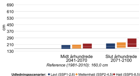
Figur 15 Højden af 20- (venstre) og 100-års (højre) stormflodhændelser for Djurslands østkyst og Anholt i fremtidsperioderne 2041-2070 og 2071-2100 under forskellige udledningsscenarier. Den grå linje viser referenceværdien for nutiden (1981-2010).
