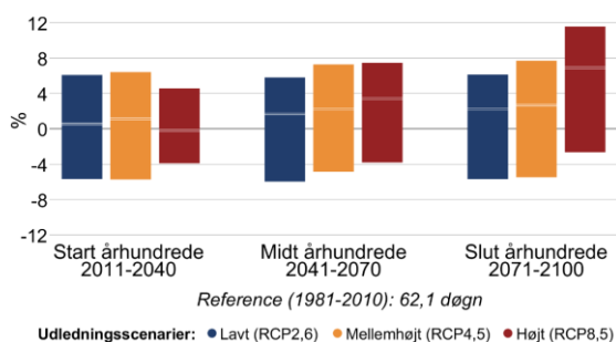
Figur 8 Procentvis ændring af tørre dage om sommeren (jun-aug) mellem 1981-2010 og fremtidsperioderne 2011-2040, 2041-2070 og 2071-2100 under forskellige udledningsscenarier i Norddjurs Kommune. Til venstre antallet af tørre dage med mindre end 1 mm nedbør, til højre længden af den længste sammenhængende tørre periode.
