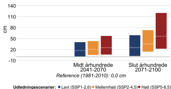
Figur 14 Ændring i middelvandstand (venstre) og hyppigheden af stormflod for Djurslands østkyst og Anholt i fremtidsperioderne 2041-2070 og 2071-2100 under forskellige udledningsscenarier. Den grå linje viser referenceværdien for nutiden (1981-2010). En stormflod defineres her som en forhøjet vandstand, der statistisk set kun forekommer én gang hvert 20. år i perioden 1981-2010. Bemærk også at denne indikator kappes ved 60 stormfloder per 20 år.
