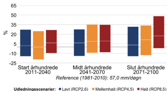
Figur 7 Procentvis ændring af ekstremnedbør hen over året mellem 1981-2010 og fremtidsperioderne 2011-2040, 2041-2070 og 2071-2100 under forskellige udledningsscenarier i Norddjurs Kommune. Til venstre 10-årshændelsen for døgnnedbør, til højre frekvensen af skybrud.
