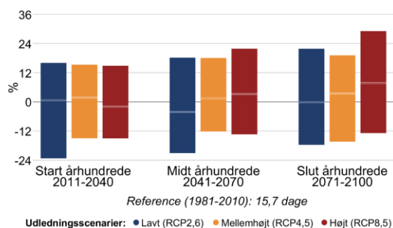
Figur 8 Procentvis ændring af tørre dage om sommeren (jun-aug) mellem 1981-2010 og fremtidsperioderne 2011-2040, 2041-2070 og 2071-2100 under forskellige udledningsscenarier i Københavns Kommune. Til venstre antallet af tørre dage med mindre end 1 mm nedbør, til højre længden af den længste sammenhængende tørre periode.
