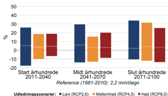
Figur 6 Procentvis ændring af middelnedbør mellem 1981-2010 og fremtidsperioderne 2011-2040, 2041-2070 og 2071-2100 under forskellige udledningsscenarier i Københavns Kommune. Til venstre sommer (jun-aug), til højre vinter (dec-feb).
