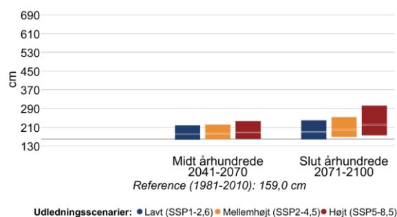
Figur 13 Højden af 20- (venstre) og 100-års (højre) stormflodhændelser for Køge Bugt i fremtidsperioderne 2041-2070 og 2071-2100 under forskellige udledningsscenarier. Den grå linje viser referenceværdien for nutiden (1981-2010).
