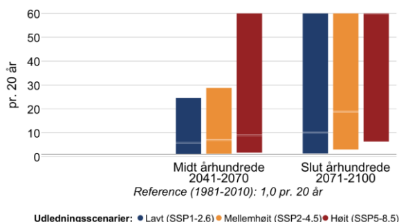
Figur 12 Ændring i middelvandstand (venstre) og hyppigheden af stormflod for Køge Bugt i fremtidsperioderne 2041-2070 og 2071-2100 under forskellige udledningsscenarier. Den grå linje viser referenceværdien for nutiden (1981-2010). En stormflod defineres her som en forhøjet vandstand, der statistisk set kun forekommer én gang hvert 20. år i perioden 1981-2010. Bemærk også at denne indikator kappes ved 60 stormfloder per 20 år.
