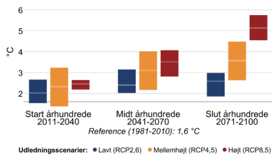
Figur 4 Gennemsnitstemperatur for sommer (jun-aug) og vinter (dec-feb) i fremtidsperioderne 2011-2040, 2041-2070 og 2071-2100 under forskellige udledningsscenarier i Københavns Kommune. Den grå linje viser referenceværdien for nutiden (1981-2010).
