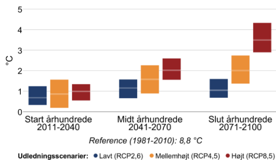
Figur 3 Ændring af gennemsnitstemperatur og antallet af hedebølgedage hen over året mellem 1981-2010 og fremtidsperioderne 2011-2040, 2041-2070 og 2071-2100 under forskellige udledningsscenarier i Københavns Kommune.
