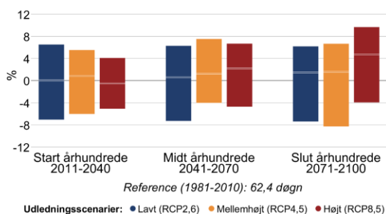
Figur 8 Procentvis ændring af tørre dage om sommeren (jun-aug) mellem 1981-2010 og fremtidsperioderne 2011-2040, 2041-2070 og 2071-2100 under forskellige udledningsscenarier i Københavns Kommune. Til venstre antallet af tørre dage med mindre end 1 mm nedbør, til højre længden af den længste sammenhængende tørre periode.
