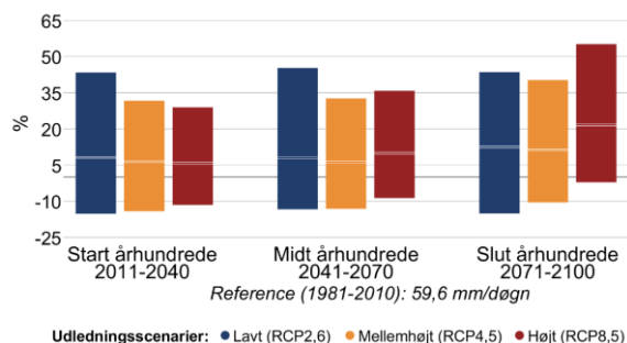
Figur 7 Procentvis ændring af ekstremnedbør hen over året mellem 1981-2010 og fremtidsperioderne 2011-2040, 2041-2070 og 2071-2100 under forskellige udledningsscenarier i Københavns Kommune. Til venstre 10-årshændelsen for døgnnedbør, til højre frekvensen af skybrud.
