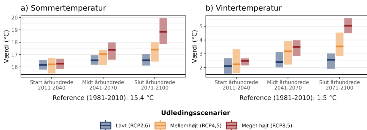
Figur 4. Fremtidens gennemsnitstemperatur for a) sommer (jun-aug) og b) vinter (dec-feb) under forskellige udledningsscenarier i Vesthimmerlands Kommune. Den sorte linje viser værdien for referenceperioden (1981-2010).
