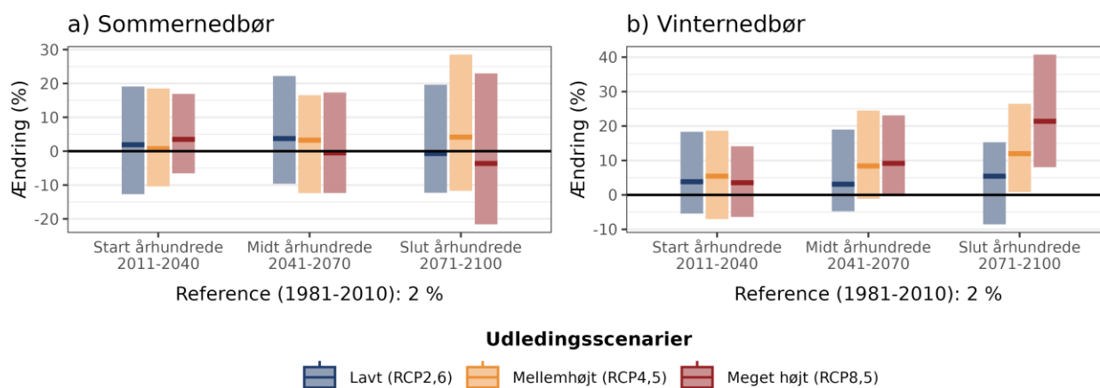
Figur 6. Procentvis ændring af middelnedbør a) om sommeren (jun-aug) og b) om vinteren (dec-feb) ift. referenceperioden 1981-2010 under forskellige udledningsscenarioer i Vesthimmerlands Kommune.
