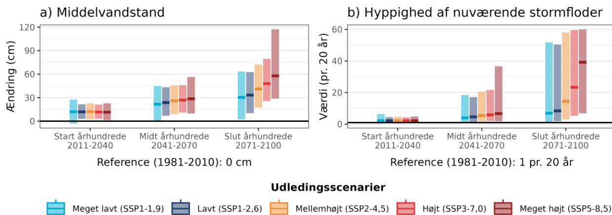
Figur 12. Fremtidens a) ændring i middelvandstand ift. referenceperioden 1981-2010 og b) hyppigheden af en nuværende 20-års stormflod for Limfjorden ved Skive under forskellige udledningsscenarier. Den sorte linje viser værdien for referenceperioden (1981-2010). Bemærk også at denne indikator maksimalt viser 60 stormfloder per 20 år, selv hvis de beregnede værdier bliver endnu højere.
