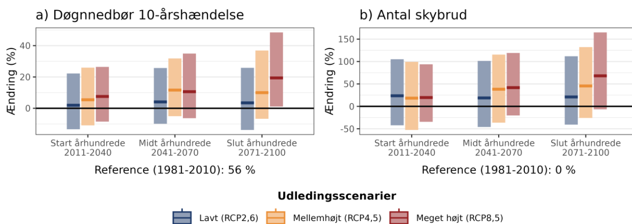
Figur 7. Procentvis ændring af a) 10-årshændelsen for døggnedbør og b) frekvensen af skybrud hen over året ift. 1981-2010 under forskellige udledningsscenarioer i Vesthimmerlands Kommune.
