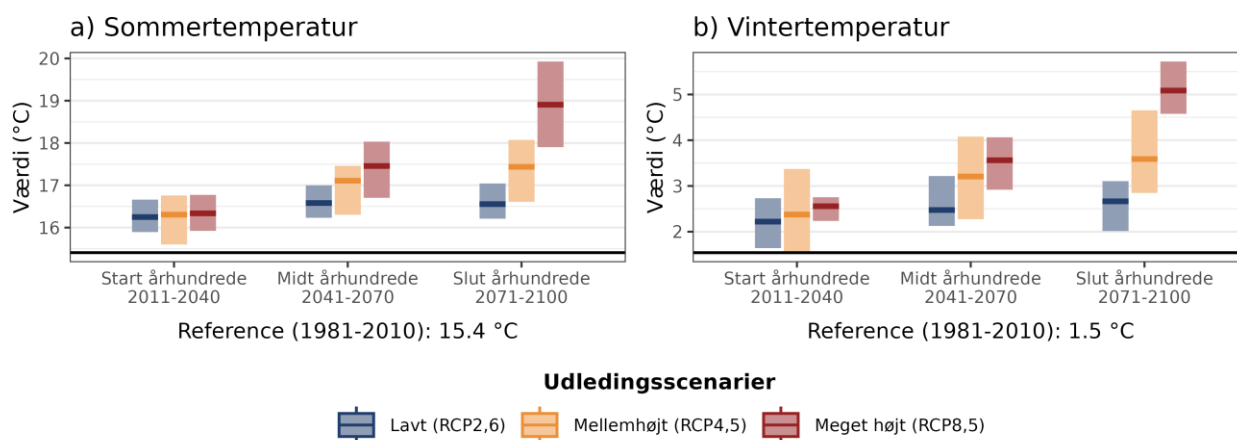
Figur 4. Fremtidens gennemsnitstemperatur for a) sommer (jun-aug) og b) vinter (dec-feb) under forskellige udledningsscenarier i Vejle Kommune. Den sorte linje viser værdien for referenceperioden (1981-2010).
