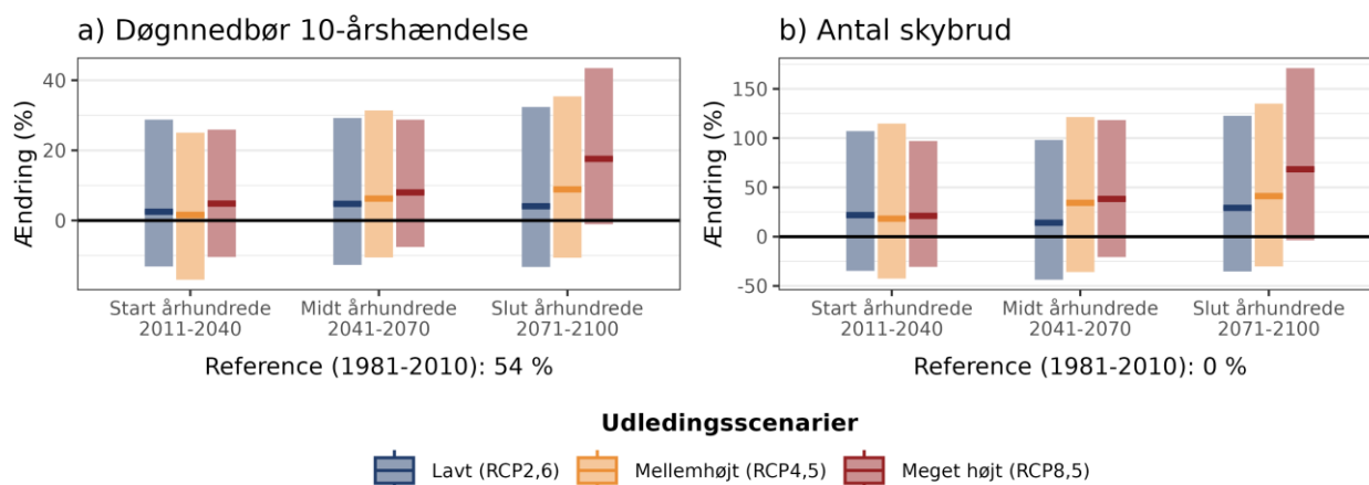
Figur 7. Procentvis ændring af a) 10-årshændelsen for døgnnedbør og b) frekvensen af skybrud hen over året ift. 1981-2010 under forskellige udledningsscenarier i Vejle Kommune.
