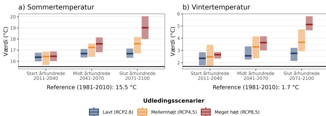
Figur 4. Fremtidens gennemsnitstemperatur for a) sommer (jun-aug) og b) vinter (dec-feb) under forskellige udledningsscenarier i Vejen Kommune. Den sorte linje viser værdien for referenceperioden (1981-2010).
