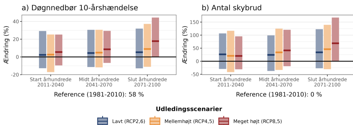
Figur 7. Procentvis ændring af a) 10-årshændelsen for døgnsnedbør og b) frekvensen af skybrud hen over året ift. 1981-2010 under forskellige udledningsscenarier i Vejen Kommune.
