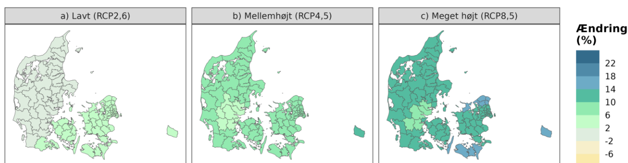
Figur 5. Den procentvise ændring mellem 1981-2010 og 2071-2100 i den gennemsnitlige mængde nedbør hen over året for hele Danmark i et a) lavt, b) mellemløjt og c) højt udledningsscenarie.
