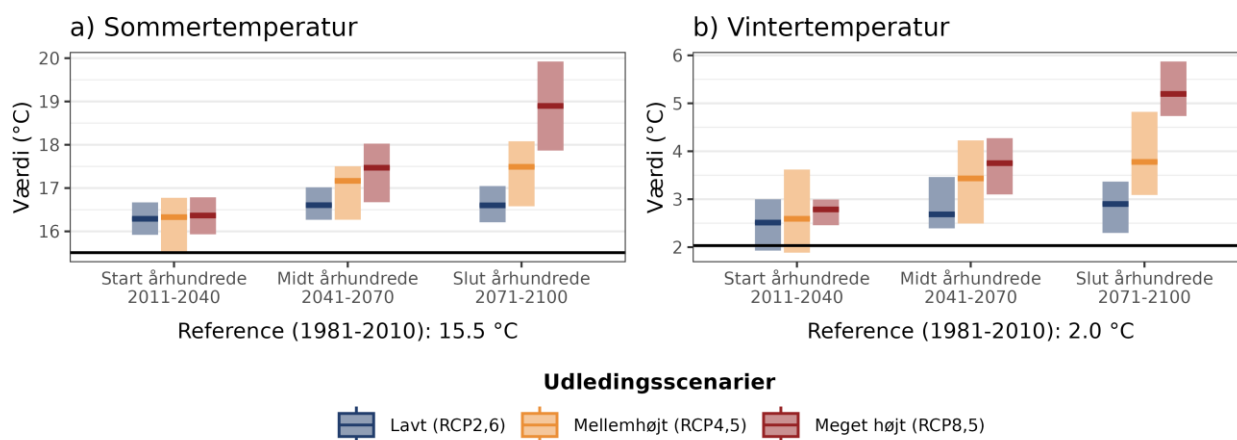
Figur 4. Fremtidens gennemsnitstemperatur for a) sommer (jun-aug) og b) vinter (dec-feb) under forskellige udledningsscenarier i Varde Kommune. Den sorte linje viser værdien for referenceperioden (1981-2010).
