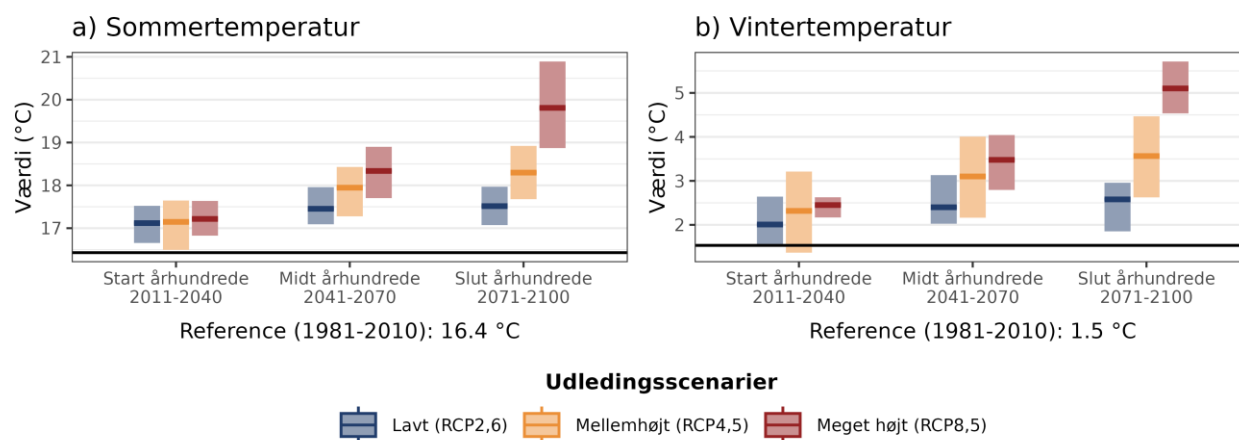
Figur 4. Fremtidens gennemsnitstemperatur for a) sommer (jun-aug) og b) vinter (dec-feb) under forskellige udledningsscenarier i Vallensbæk Kommune. Den sorte linje viser værdien for referenceperioden (1981-2010).
