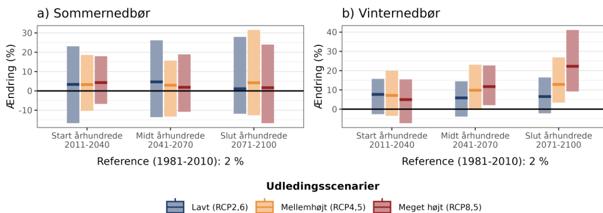
Figur 6. Procentvis ændring af middelnedbør a) om sommeren (jun-aug) og b) om vinteren (dec-feb) ift. referenceperioden 1981-2010 under forskellige udledningsscenarioer i Vallensbæk Kommune.
