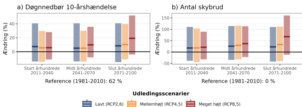
Figur 7. Procentvis ændring af a) 10-årshændelsen for døggnedbør og b) frekvensen af skybrud hen over året ift. 1981-2010 under forskellige udledningsscenarioer i Vallensbæk Kommune.
